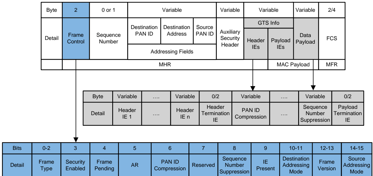
图 4. IEEE 802.15.4 General MAC Frame Format
