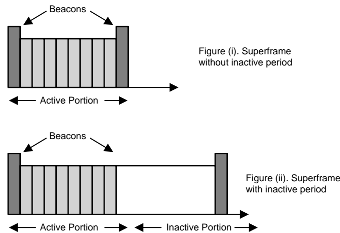
图 5. Beacon Frame Structure
