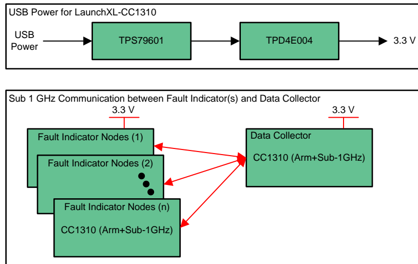
图 1. TIDA-00816 Block Diagram
