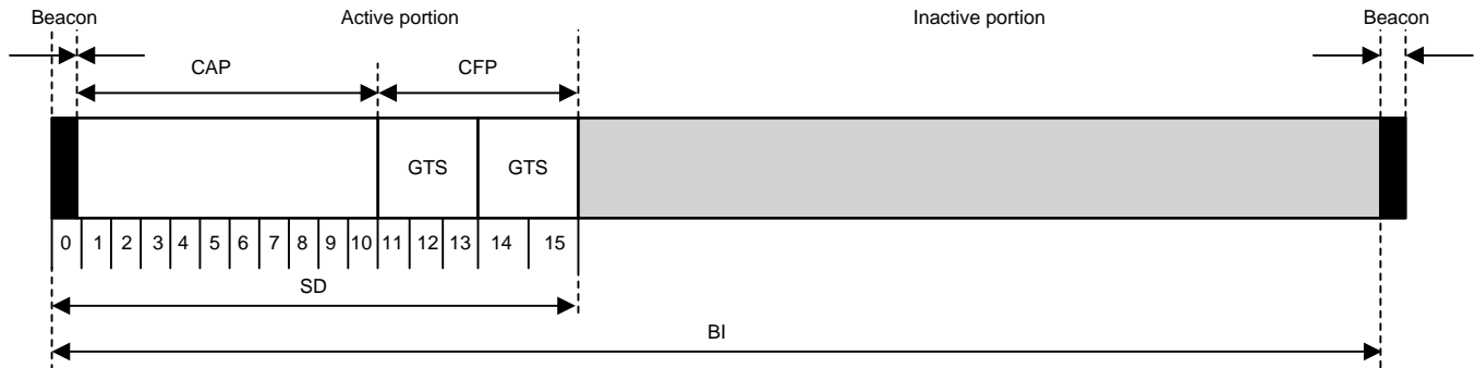
图 7. IEEE 802.15.4 Superframe Structure
