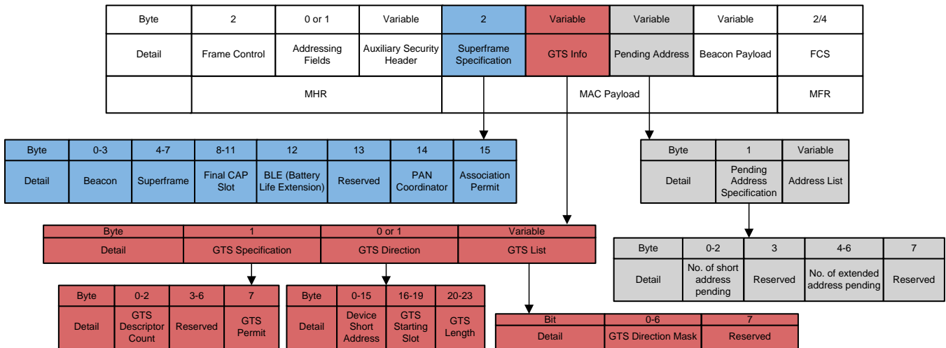
图 8. IEEE 802.15.4 Beacon Frame Format
