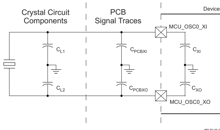
图 6-18. 负载电容
