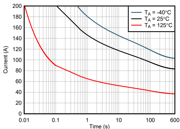
图 8-2. Short-Circuit Duration
