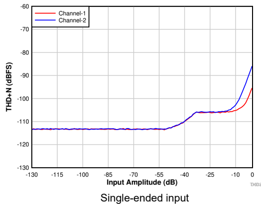
图 7-6. THD+N vs Input Amplitude With DRE Enabled
