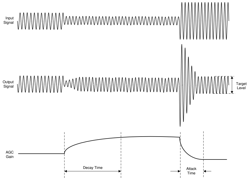
图 8-63. AGC Characteristics
