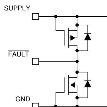
图 7-17. FAULT Pin
