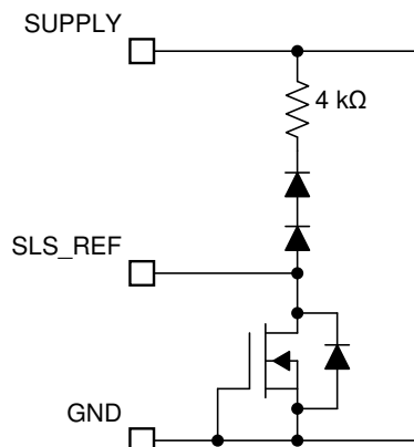
图 7-23. SLS_REF Pin
