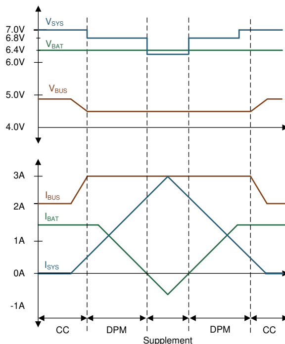
图 9-8. DPM Response
