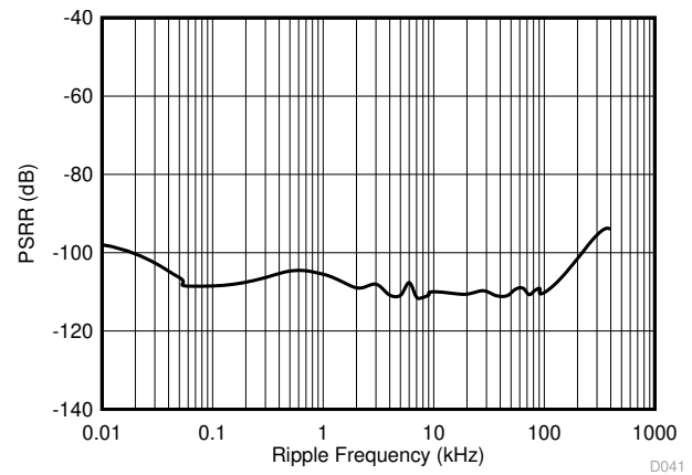
图 6-30. 电源抑制比与纹波频率间的关系
