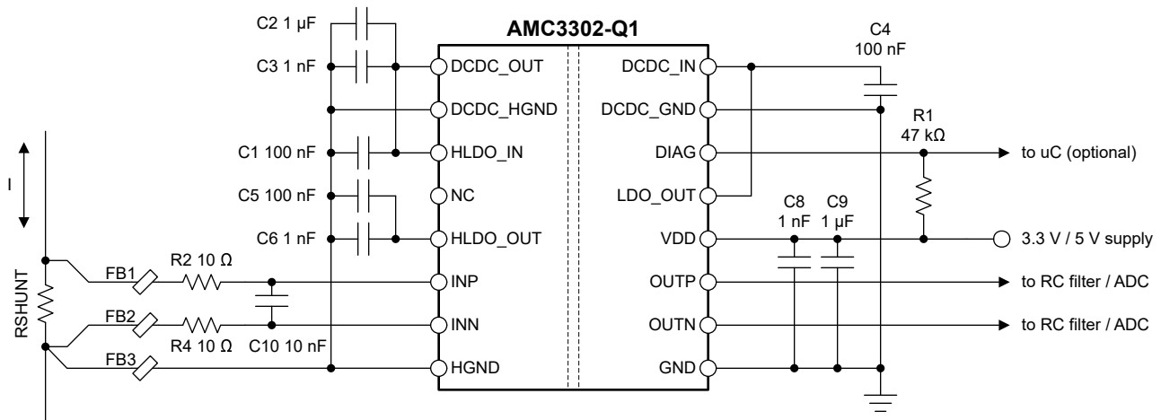
图 9-1. 解耦 AMC3302-Q1
