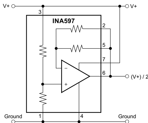
图 9-7. 伪接地发生器
