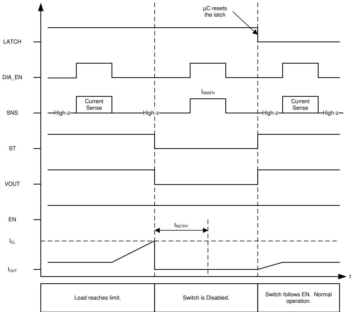
图 8-5. 电流限制 - 版本 A、B、E - 锁存行为
