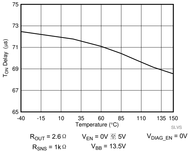
图 6-9. 导通延迟时间 ( t_{DR} ) 与温度间的关系
