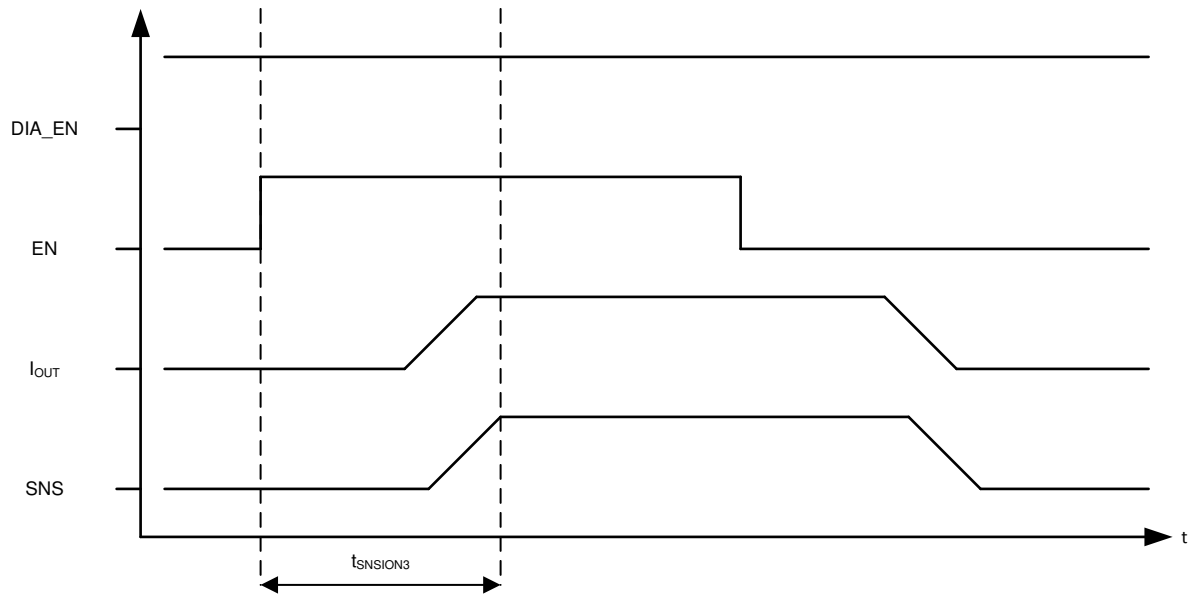
图 8-13. 低占空比应用中的电流检测
