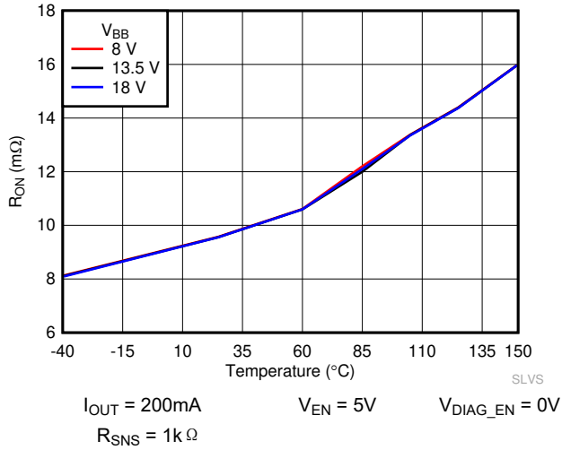
图 6-7. 导通电阻 ( R_{ON} ) 与温度间的关系
