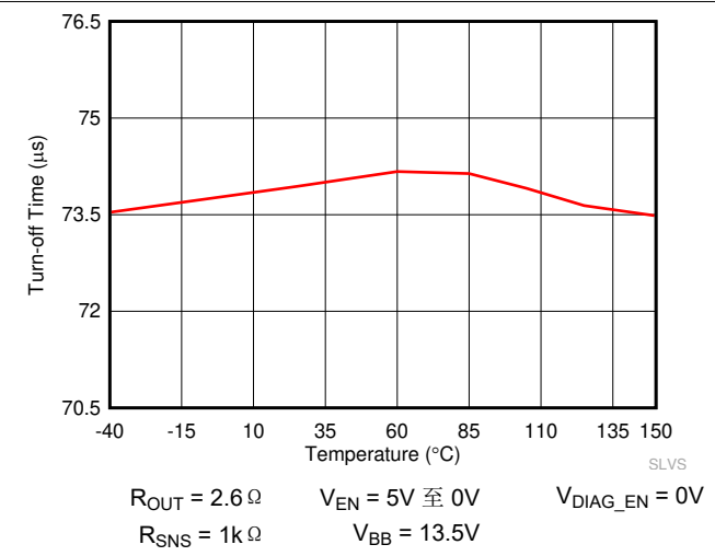
图 6-14. 关断时间 ( t_{OFF} ) 与温度间的关系
