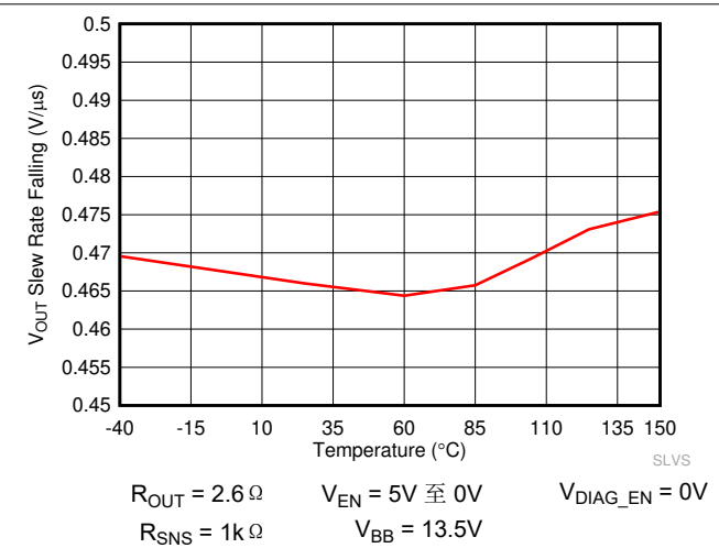
图 6-12. V_{OUT} 转换率下降 ( SR_F ) 与温度间的关系
