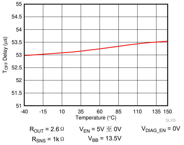
图 6-10. 关断延迟时间 ( t_{DR} ) 与温度间的关系
