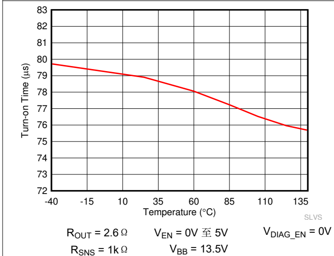
图 6-13. 导通时间 ( t_{ON} ) 与温度间的关系
