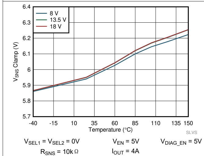
图 6-21. 感应引脚钳位电压 ( V_{SNSCLAMP} ) 与温度间的关系
