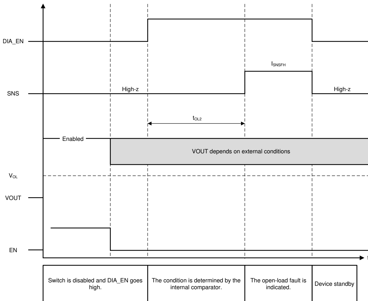
图 8-11. 开路负载
