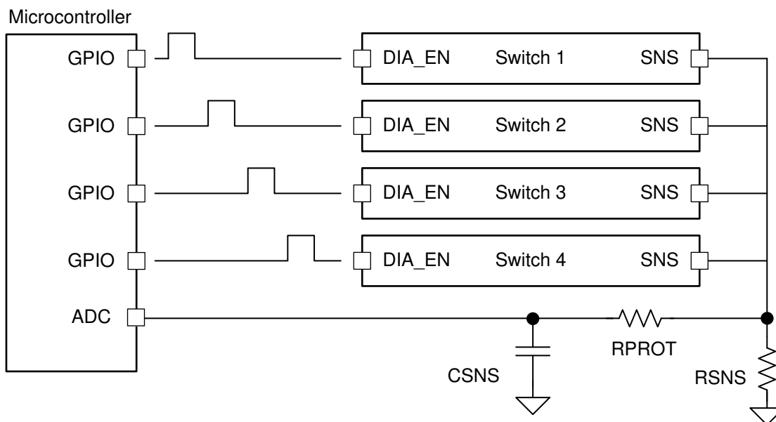
图 8-12. 在多个器件之间共享 R_{SNS}
