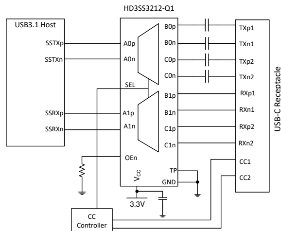
简化原理图
