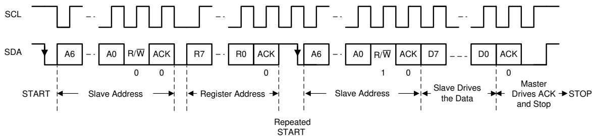
图 6-19. I 2 C 接口 READ 从 TPS650861 在 F/S 模式 (仅支持重复 START)
