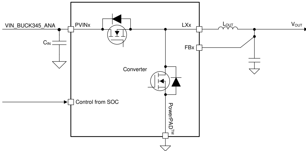
图 7-3. Converter Diagram
