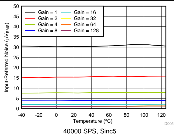
图 20. Noise vs Temperature
