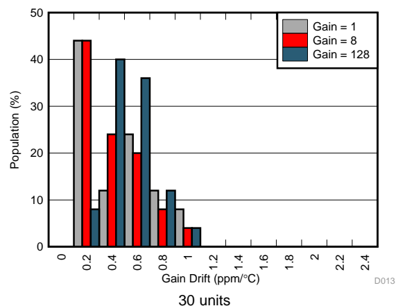
图 16. Gain Error Drift Distributions
