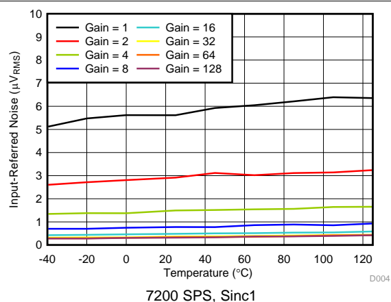
图 19. Noise vs Temperature
