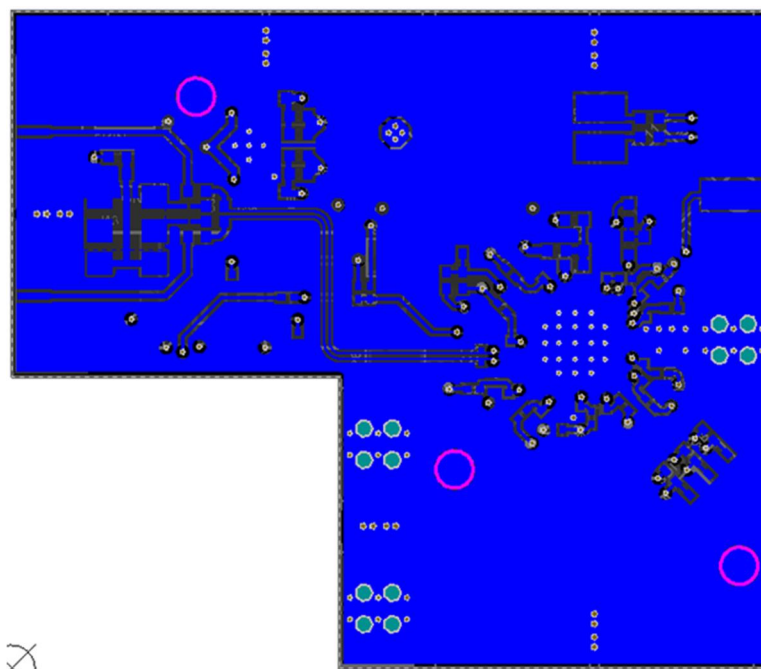
图 99. Bottom Layer
