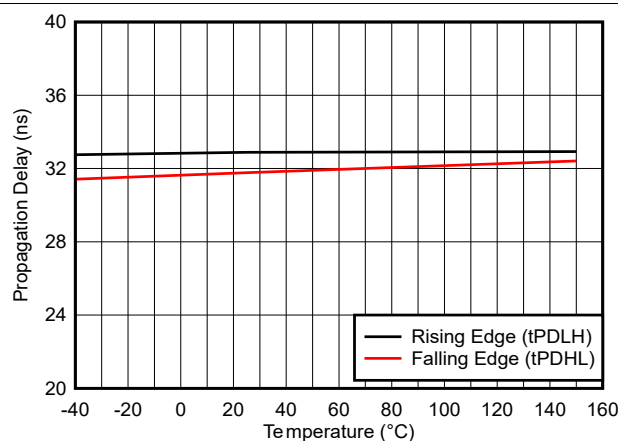
图 5-12. 传播延迟与温度之间的关系
