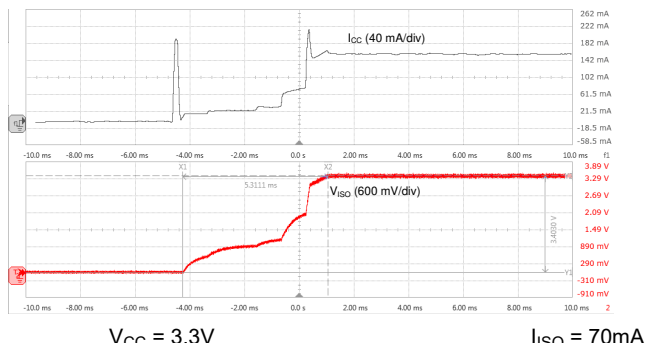
V_{CC} = 3.3V I_{ISO} = 70mA 输入电流尖峰是为输入电源去耦电容器充电而造成的。
