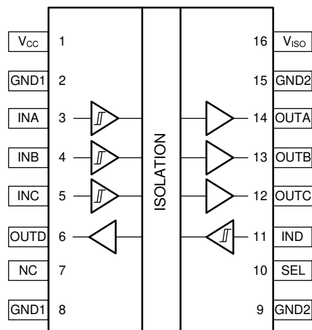
图 6-2. ISOW7841 DWE 封装 16 引脚 SOIC-WB 顶视图
