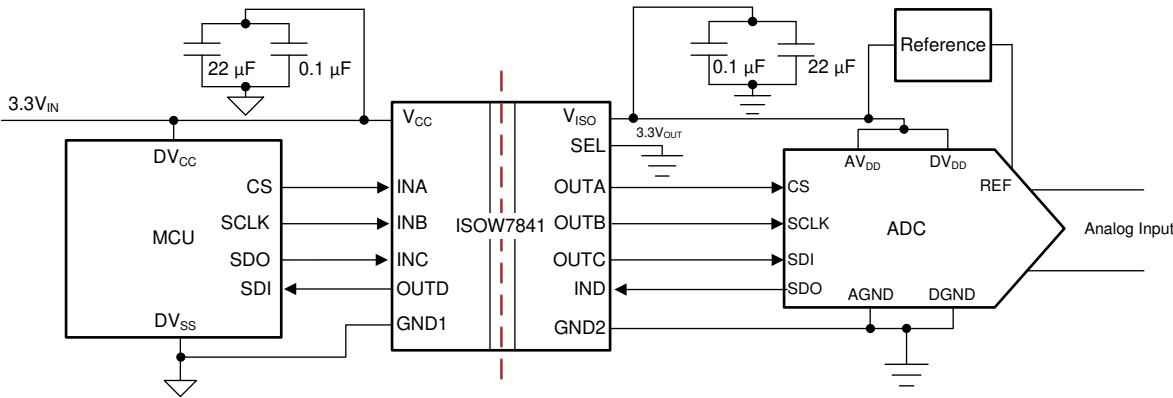
图 10-1. 采用 ISOW7841
