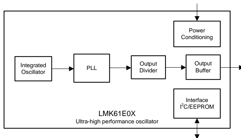
引脚分布和简化框图
