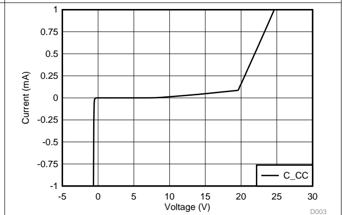
图 24. C_CC IV Curve
