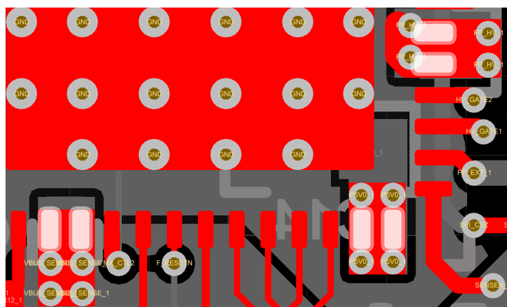
图 12-7. Top Polygonal Pours
