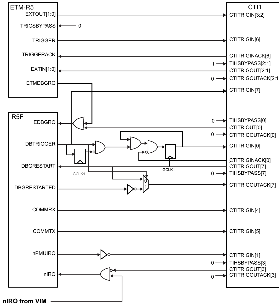
图 6-25. CTI1 Mapping
