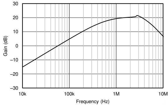
图 6-8. LNA 增益与频率之间的关系
