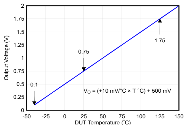
全量程摄氏温度传感器 ( -40^{\circ}\text{C} 至 125^{\circ}\text{C} )
