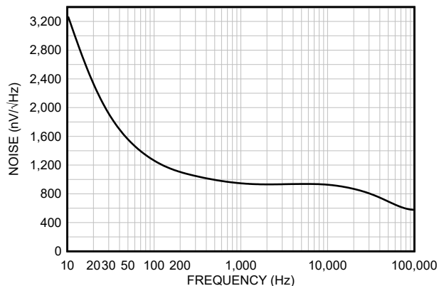
图 6-16. 噪声电压 (新芯片)
