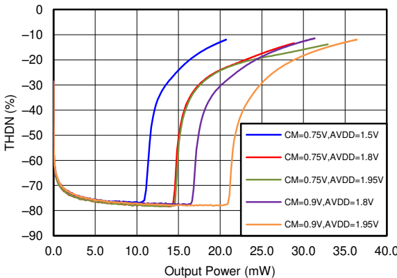
图 9-2. 总谐波失真 + 噪声与 4 Ω 扬声器功率间的关系
