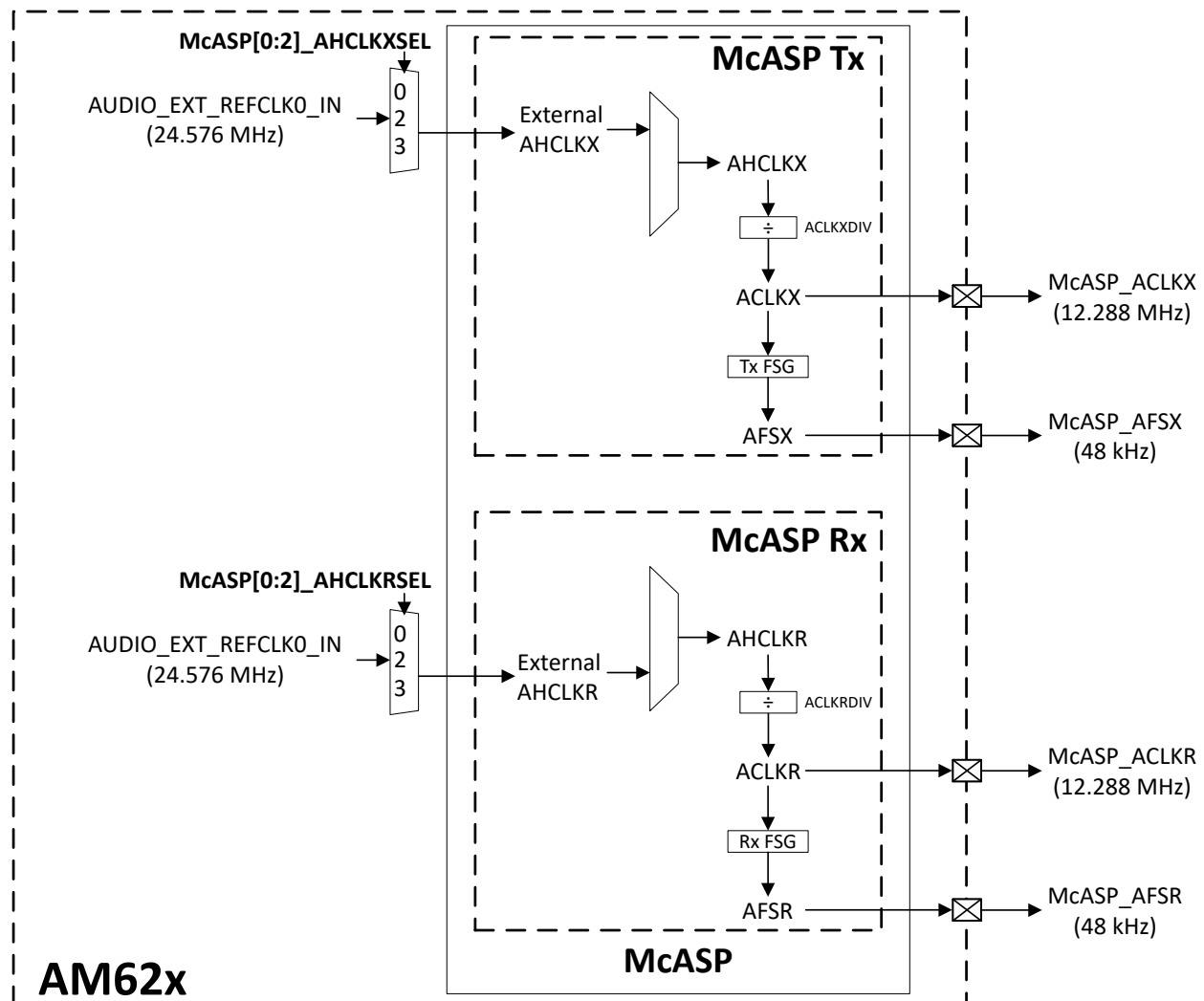
图 3-4. 具有 AUDIO_EXT_REFCLK0 AHCLK 基准的 McASP 时钟控制器
