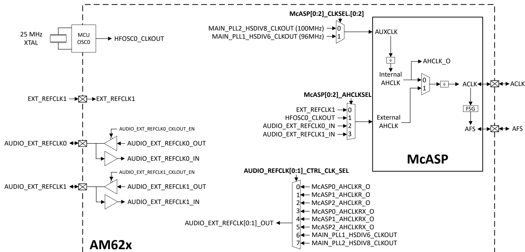
图 3-1. AM62x McASP 连接
