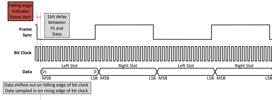
图 1-2. I2S 时序图
