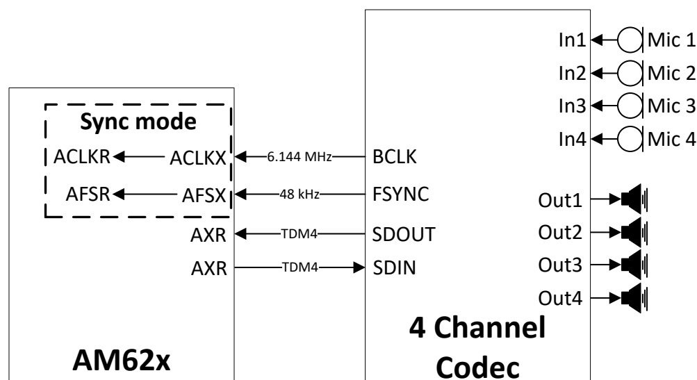
图 5-2. 同步模式下 McASP 作为时钟外设的编解码器回放
