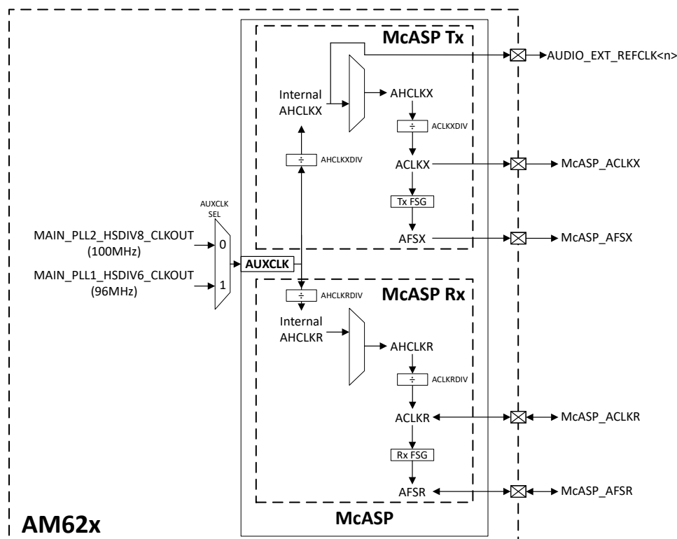
图 3-3. 具有 AUXCLK 源的 McASP 控制器
