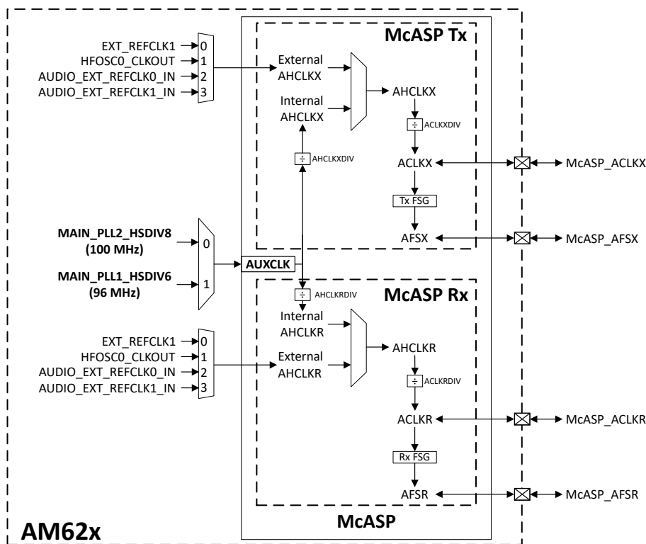
图 3-2. McASP 详细介绍
