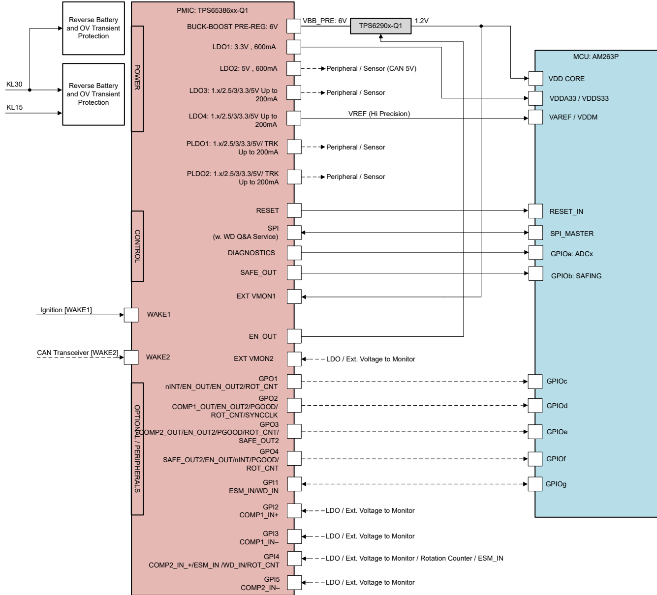
图 2-1. TIPA-050072 电源连接
