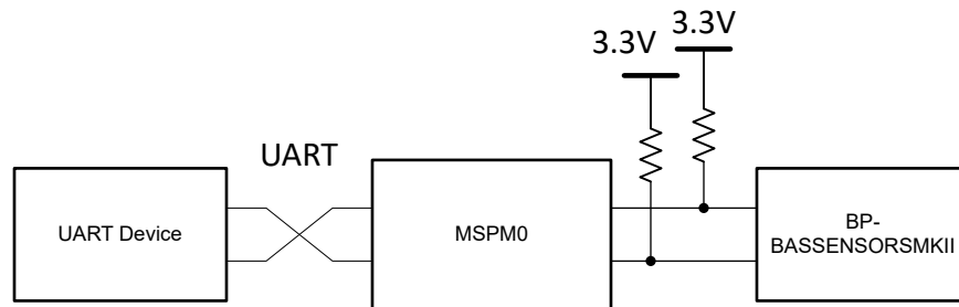
图 1-1. 系统功能方框图
