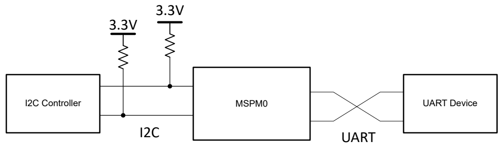
图 1-1. 系统功能方框图
