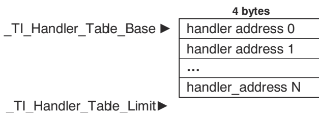
图 18-1. 处理程序表格式
