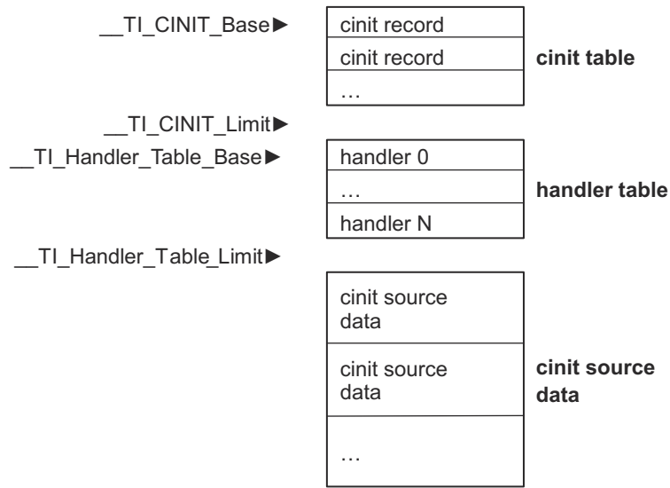
图 18-4. .cinit 段
