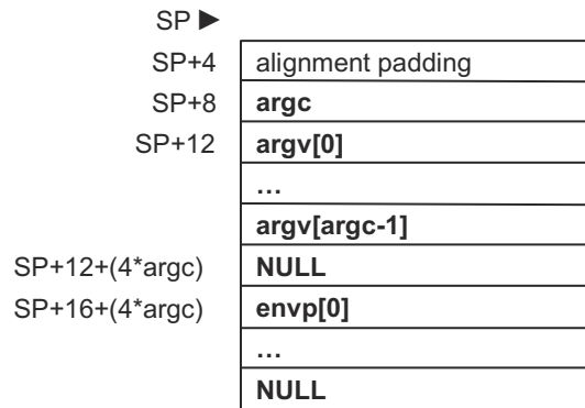
图 15-1. 程序加载映射数据结构中的栈初始内容
