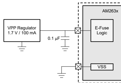
图 2-19. AM26x 电子保险丝 VPP - 外部电源实施
