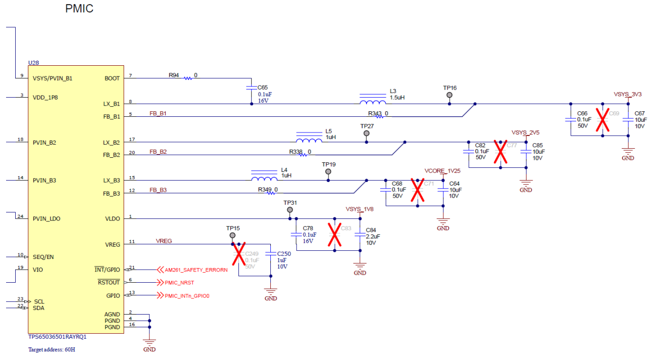
图 2-6. LP-AM261 PMIC 实施
