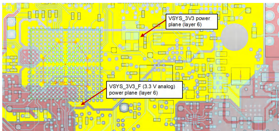
图 2-15. AM263x LaunchPad PDN 仿真 - 3.3V 数字和模拟 I/O 电源仿真域 (A)
