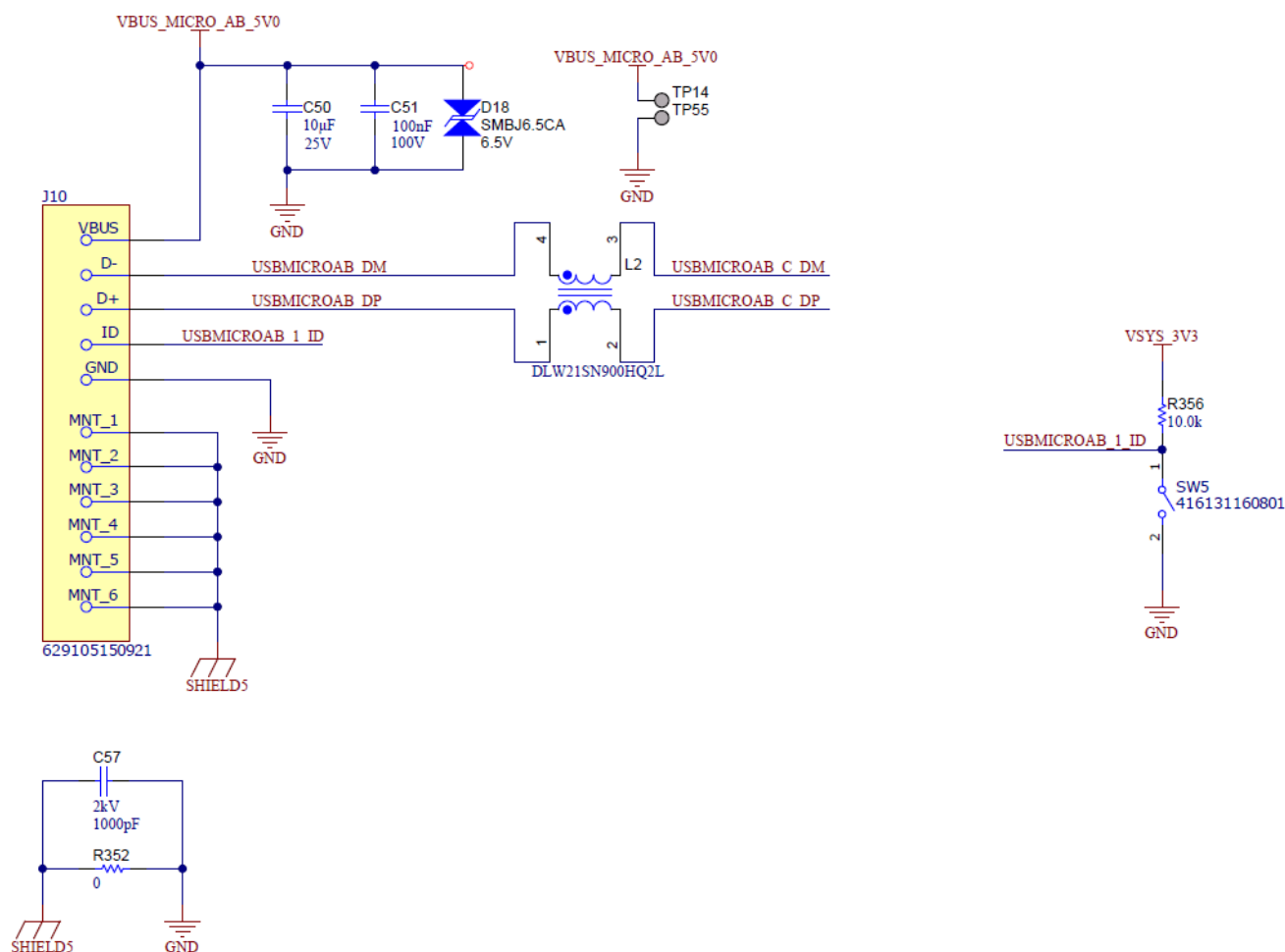
图 8-1. 显示关键信号的 USB 2.0 Micro-AB 端口 - LP-AM261
