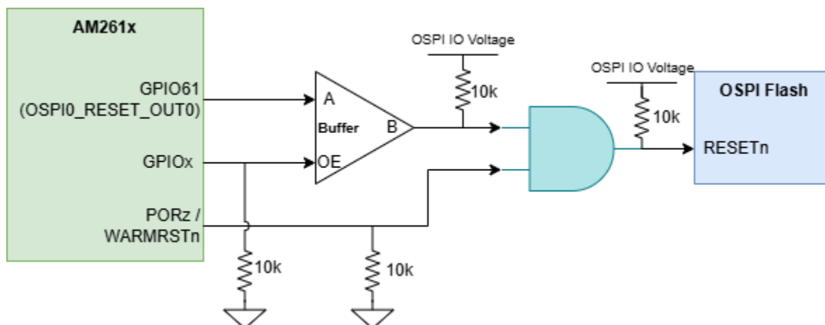
图 6-9. 使用缓冲后的 GPIO61 和 PORz、WARMRESETn 来复位 OSPI 闪存
