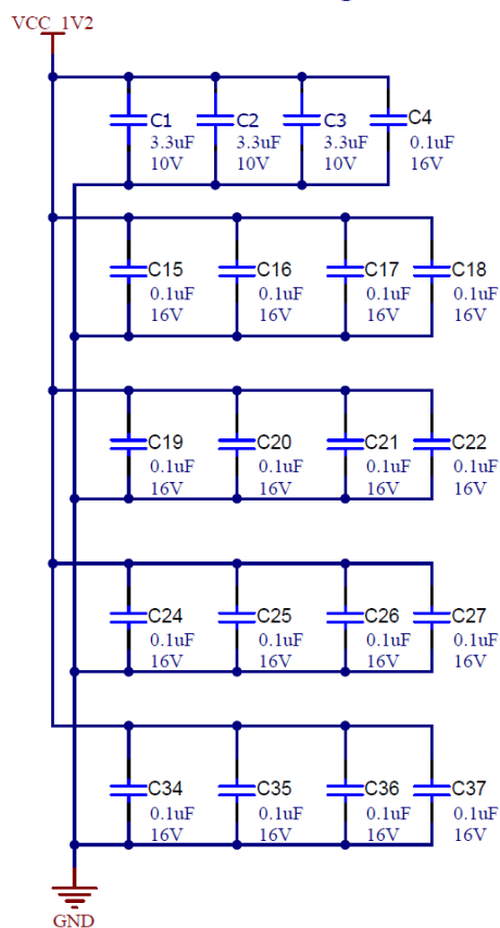
图 2-7. AM263x LaunchPad 摘录 - 1.2V 电源去耦原理图
