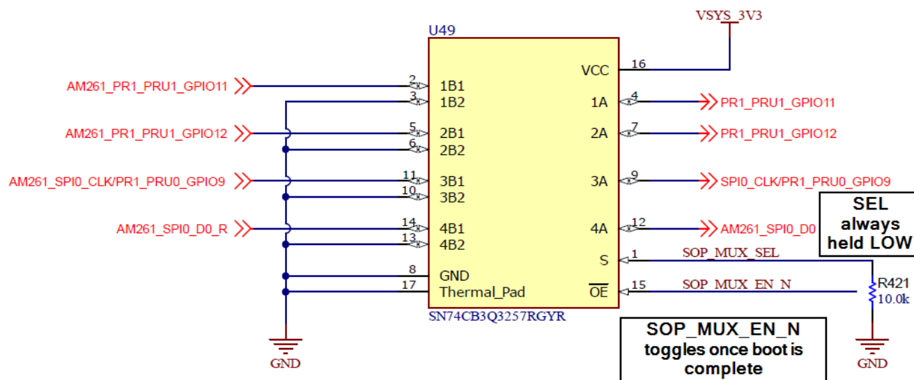
图 5-5. LP-AM261 SOP 隔离多路复用器
