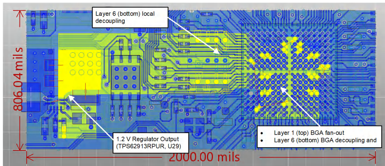
图 2-13. AM263x LaunchPad PDN 仿真 - 1.2V 内核电源仿真域
