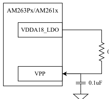
图 2-20. AM263Px/AM261x 电子保险丝 VPP - 内部模拟 LDO 实现
