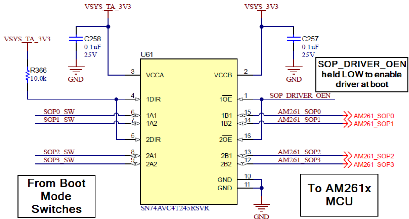
图 5-7. LP-AM261 SOP 状态驱动器
