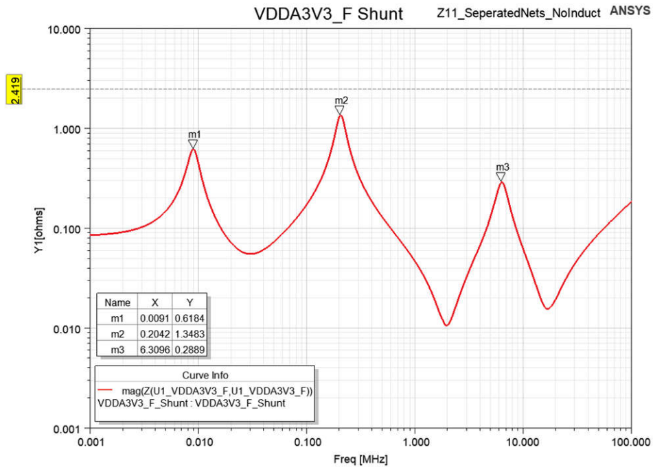
图 2-18. AM263x LaunchPad PDN 仿真 - 3.3V 模拟 I/O 电源仿真 Z11
