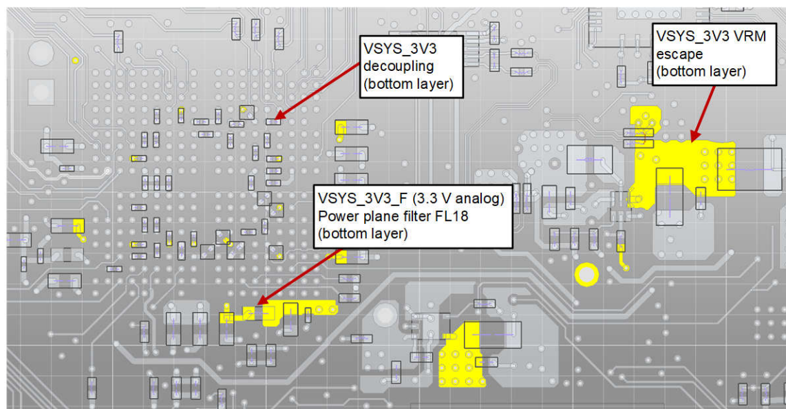
图 2-16. AM263x LaunchPad PDN 仿真 - 3.3V 数字和模拟 I/O 电源仿真域 (第 8 层，底部)
