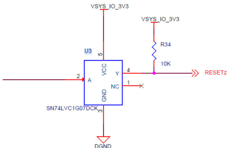
图 4-5. AM263x 控制卡原理图摘录 - WARMRSTn 按钮开漏驱动器
