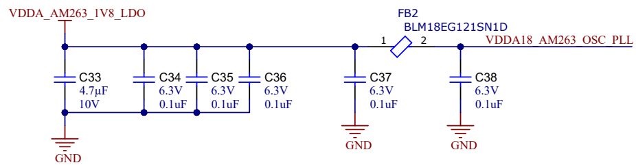
图 2-9. AM263x LaunchPad 摘录 - 1.8V 数字 I/O 和模拟 I/O 去耦和滤波原理图
