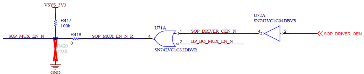
图 5-8. LP-AM261 SOP 隔离多路复用器输出使能生成
