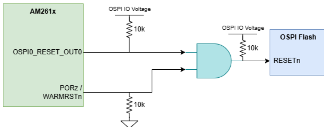
图 6-8. 使用 OSPI0_RESET_OUT0 和 PORz、WARMRESETn 复位 OSPI 闪存
