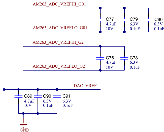
图 2-10. AM263x LaunchPad 摘录 - ADC 和 DAC VREF 去耦原理图
