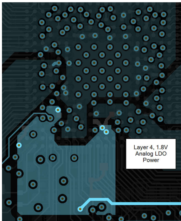
图 14-28. AM261x LaunchPad 摘录 - 1.8V 模拟电源过孔扇出和平面布线，第 4 层
