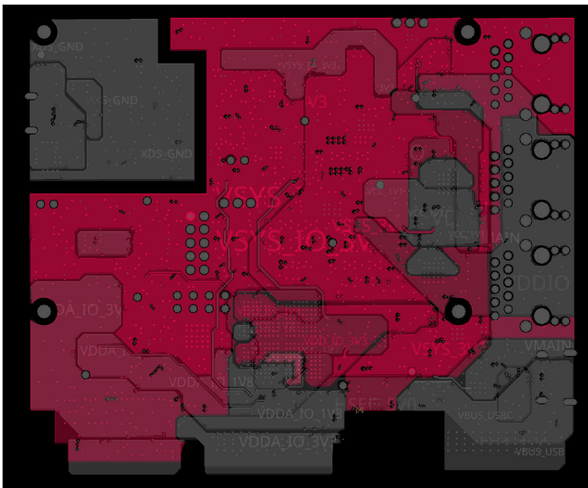
图 14-12. AM263x controlCARD 摘录 - 第 5 层和第 6 层上的 3.3V 数字和模拟电源平面
