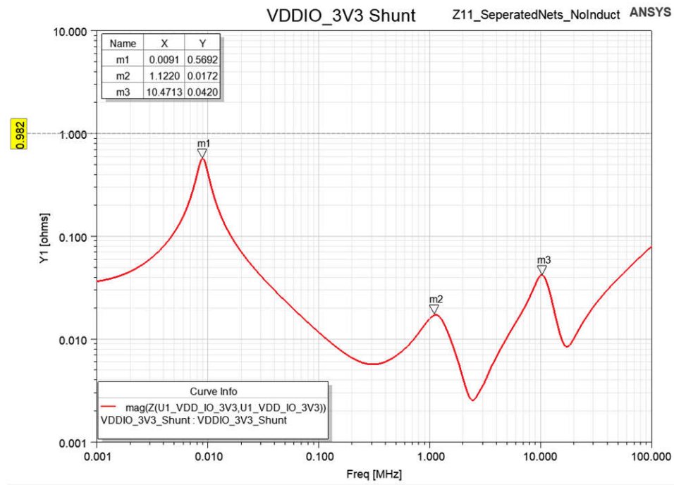
图 2-17. AM263x LaunchPad PDN 仿真 - 3.3V 数字 I/O 电源仿真 Z11
