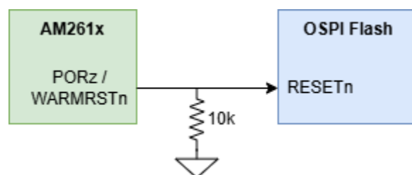
图 6-7. 使用 PORz 或 WARMRESETn 复位 OSPI 闪存
