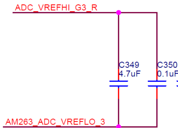
图 2-11. AM263Px controlCard 摘录 - 其他 VREFHI_G3 和 VREFLO_G3 连接
