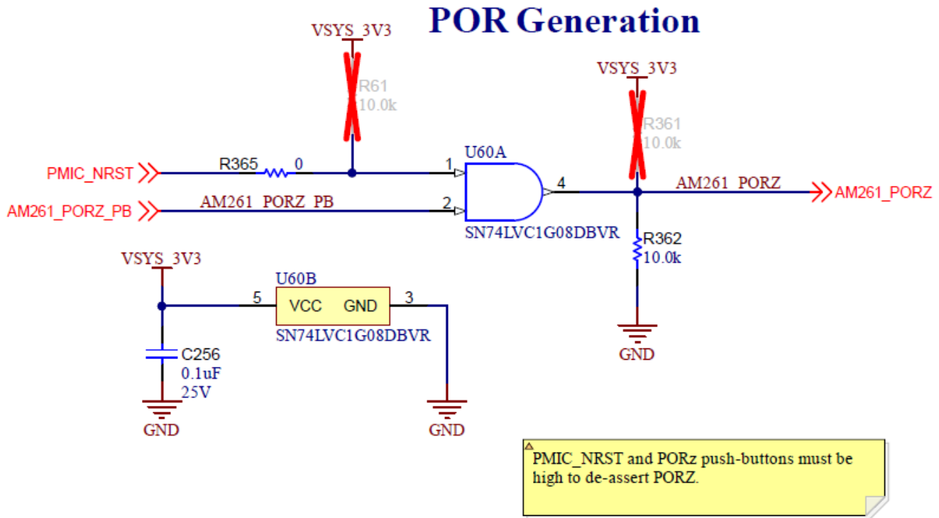
图 4-3. AM261x LaunchPad 原理图摘录 - PORz 的生成
