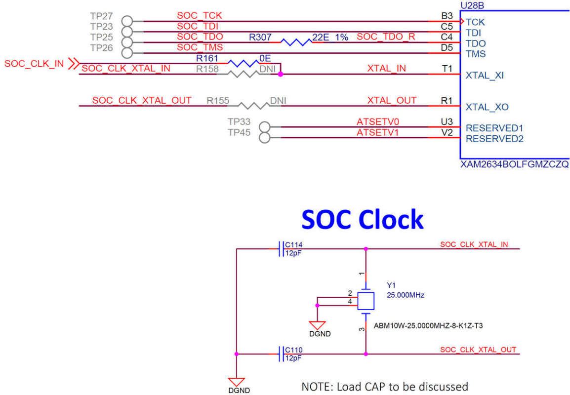
图 3-1. AM263x 控制卡原理图摘录 ( 针对完整的晶体和振荡器输入要求 )
