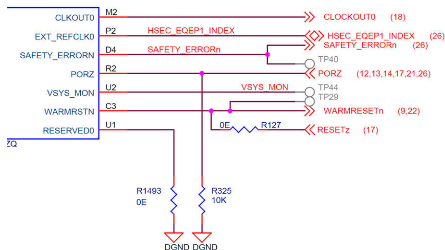
图 4-4. AM263x 控制卡原理图摘录 - PORz 和 WARMRSTn 引脚排列
