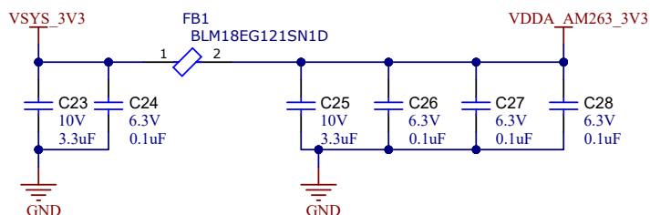
图 2-8. AM263x LaunchPad 摘录 - 3.3V 数字 I/O 和模拟 I/O 去耦和滤波原理图
