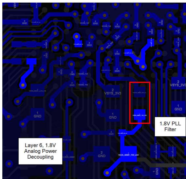
图 14-29. AM261x LaunchPad 摘录 - 第 6 层上的 1.8V 模拟电源去耦
