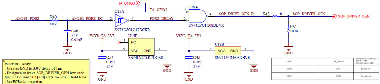
图 5-6. LP-AM261 PORz SOP 驱动器 RC 延迟
