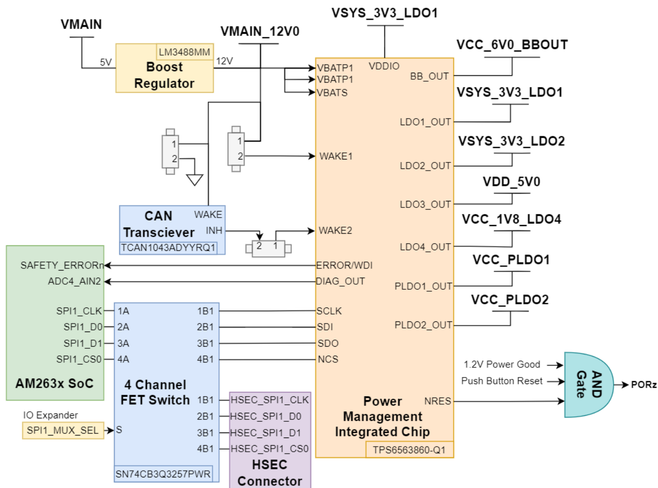
图 2-5. AM263Px TMDSCNCD263P PMIC 实现
