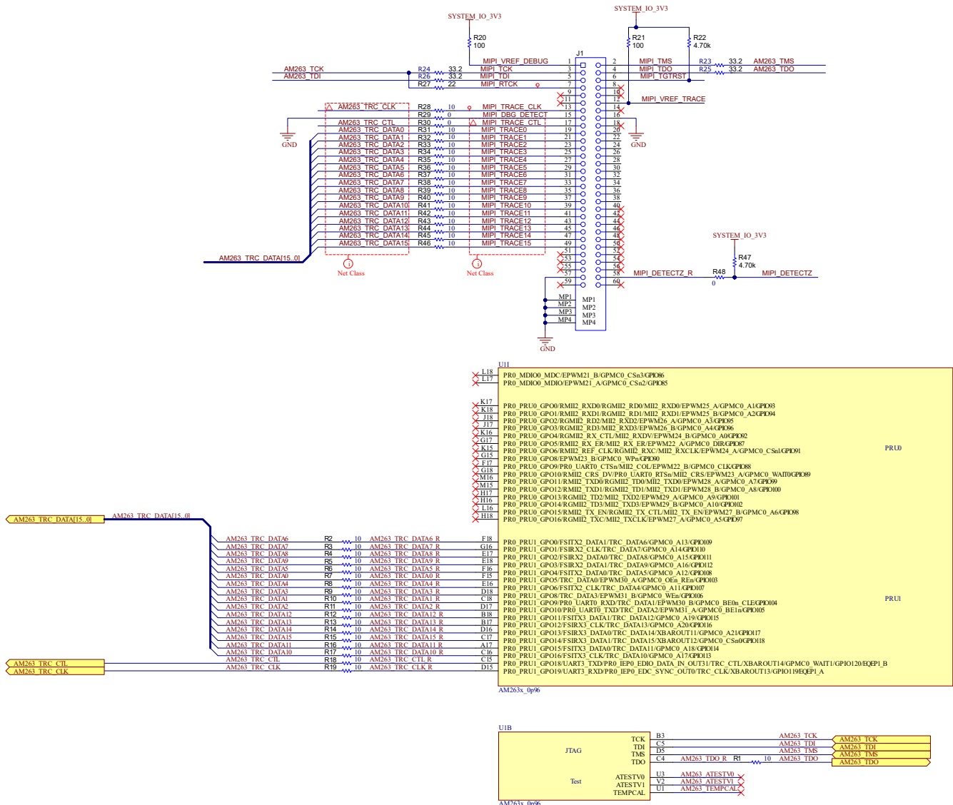
图 7-1. MIPI-60 JTAG 和 16 位跟踪实施示例
