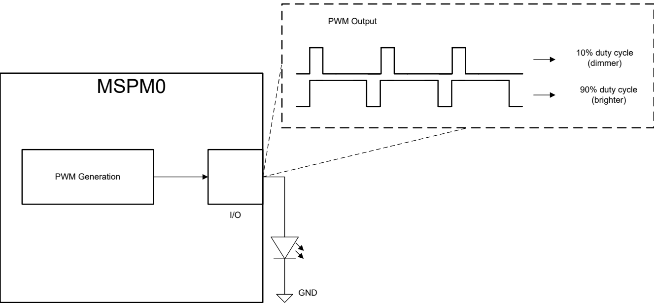
图 1-1. 子系统功能方框图
