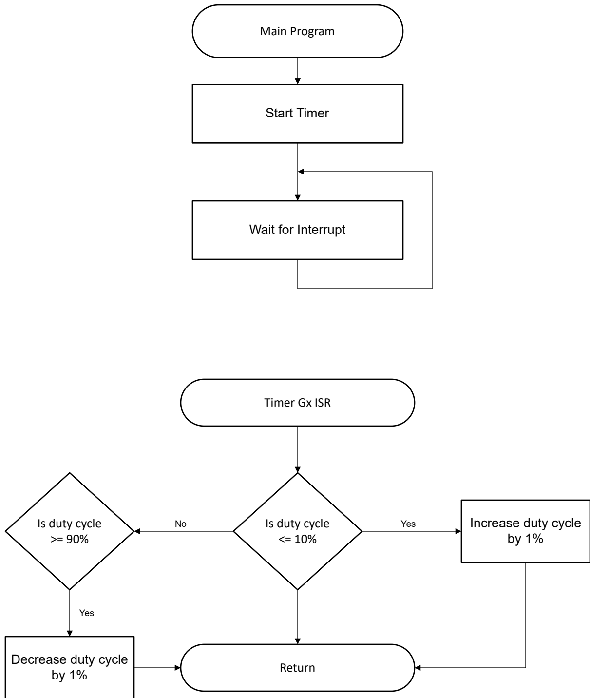
图 1-2. 应用软件流程图
