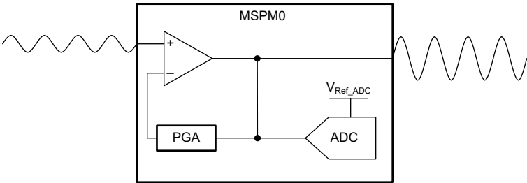
图 1-1. 子系统功能方框图
