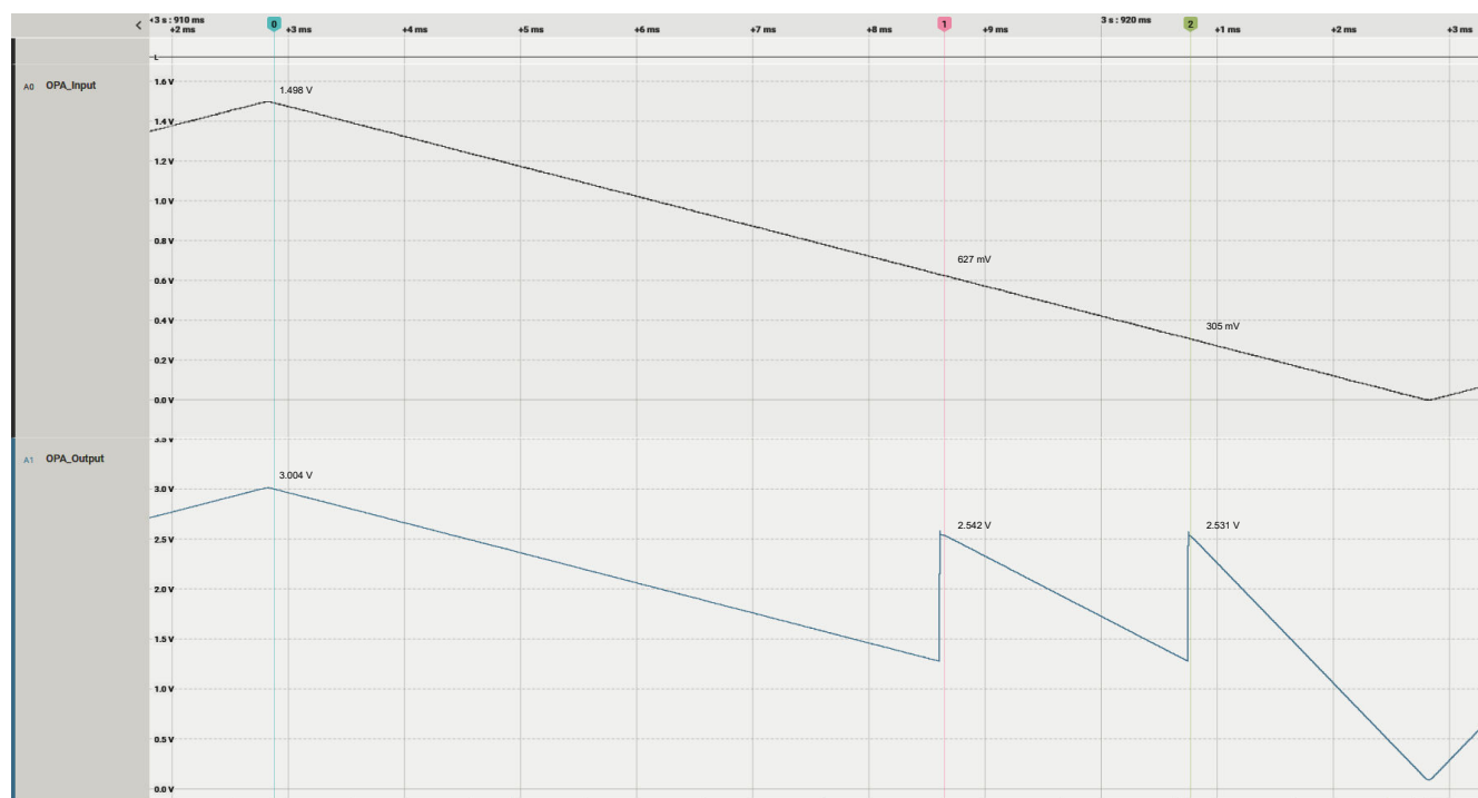
图 1-4. 减小 OPA PGA 增益
