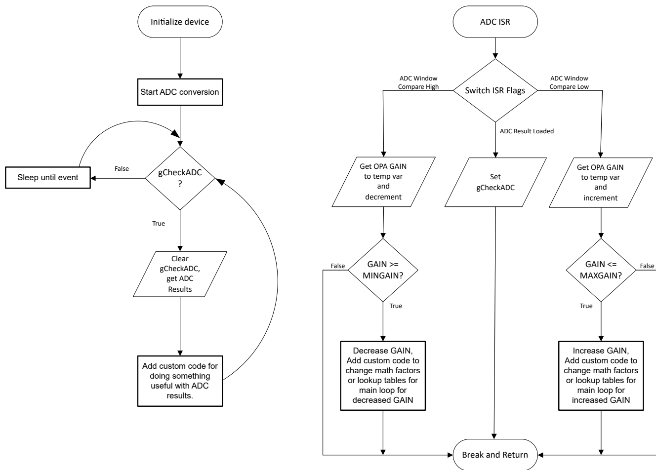
图 1-2. 应用软件流程图
