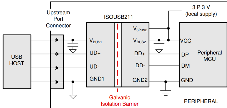
示例：为 USB 2.0 接口系统提供高电压保护和增强的信号完整性
