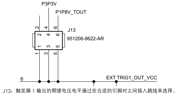
图 3: J13 的原理图
