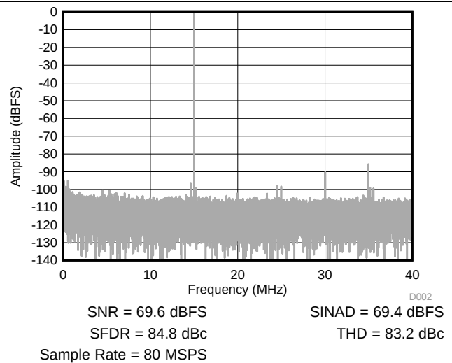
图 5. FFT for 15-MHz Input Signal
