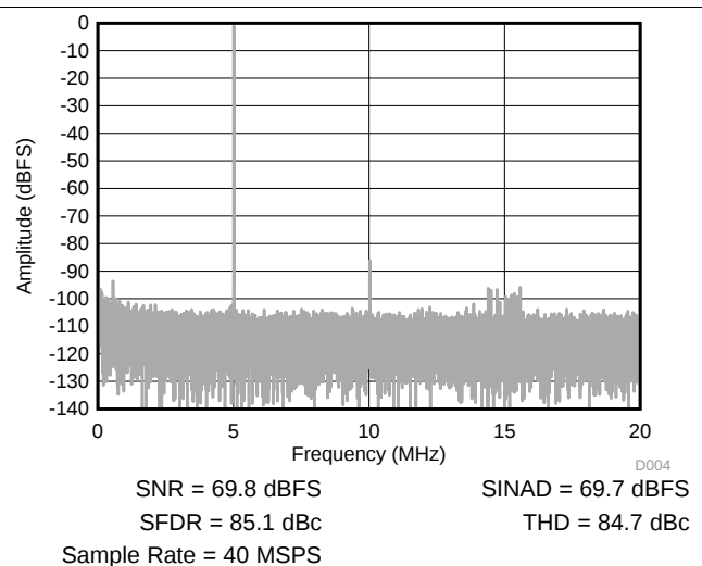
图 7. FFT For 5-MHz Input Signal
