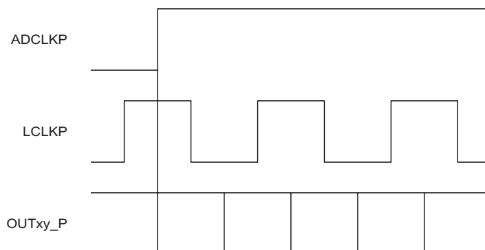
图 46. LCLK Default Phase (PHASE_DDR[1:0] = 10)
