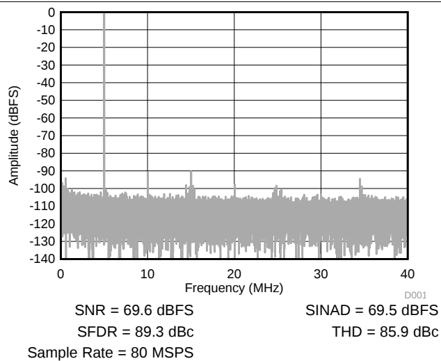
图 4. FFT for 5-MHz Input Signal
