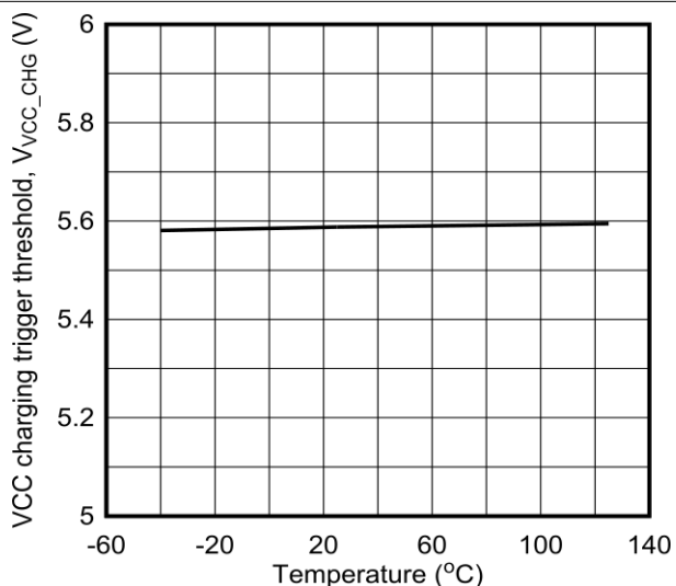
图 6-4. VCC 充电触发电压与结温间的关系
