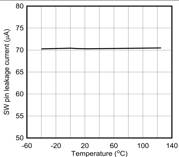
图 6-6. SW 引脚漏电流与结温间的关系
