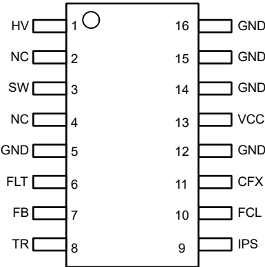
图 5-2. UCG2883x/4x 16 引脚 SOIC ( 顶视图 )
