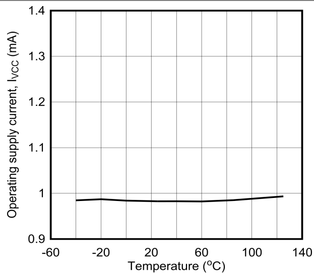
图 6-5. 工作电源电流与结温间的关系
