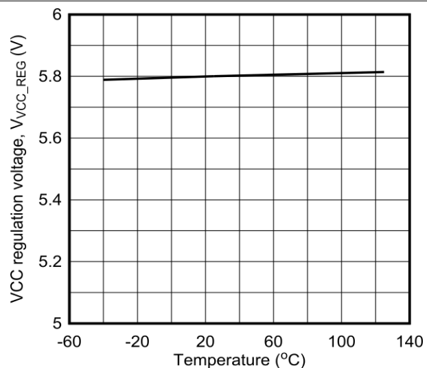
图 6-3. VCC 稳压电压与结温间的关系
