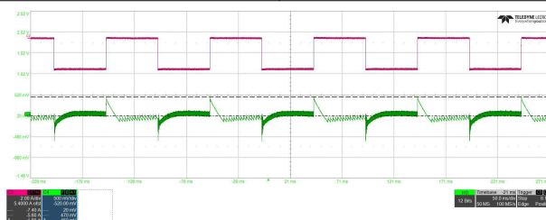
图 8-9. 230VAC 和 20V 输出时的负载瞬态
