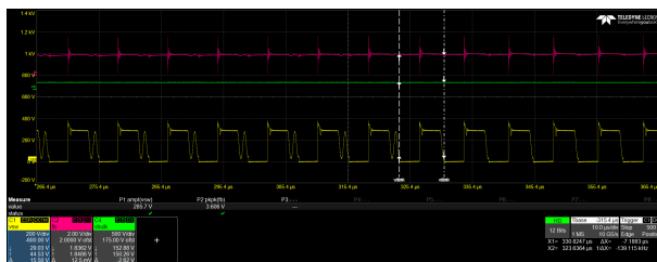
图 8-2. 115VAC 时的第一个谷底和第二个谷底运行
