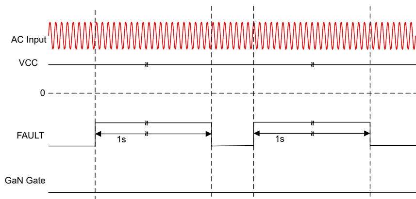
图 7-12. 自动重试故障响应
