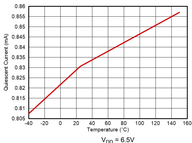
图 5-5. 静态电流
