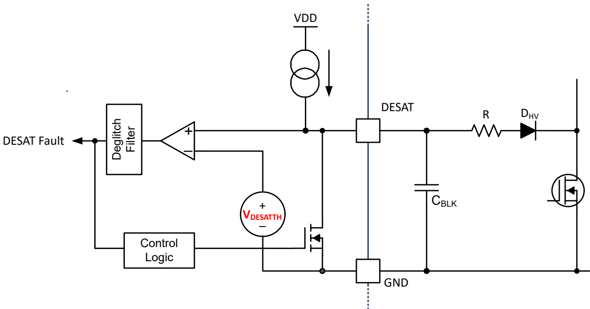
图 6-3. DESAT 保护
