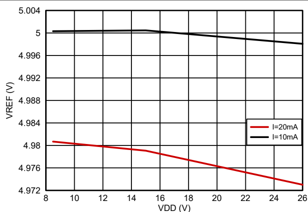
图 5-20. V_{REF} 电压与 V_{DD} 间的关系
