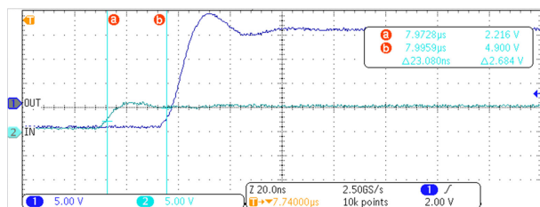
图 7-3. UCC57102Z 上升 ( 导通 ) 传播延迟
