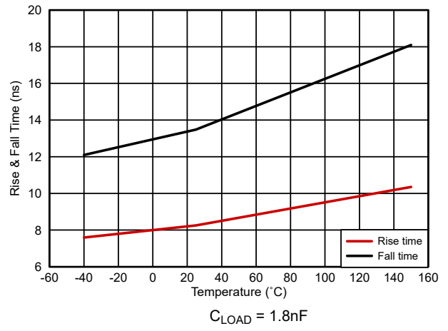
图 5-16. 输出上升和下降时间
