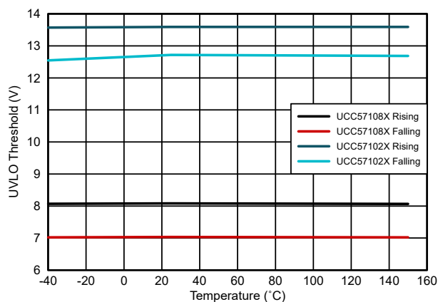
图 5-9. UVLO 阈值
