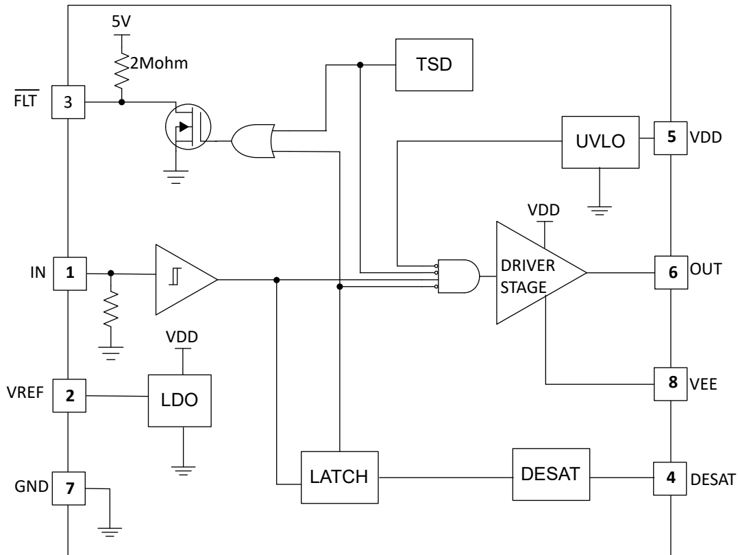
图 6-1. UCC57102Z 简化功能方框图
