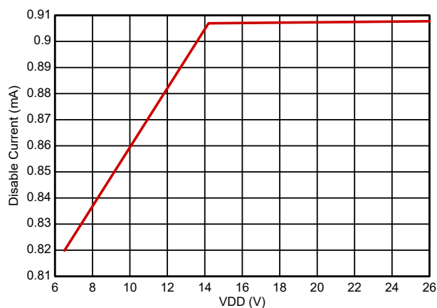
图 5-7. 禁用电流
