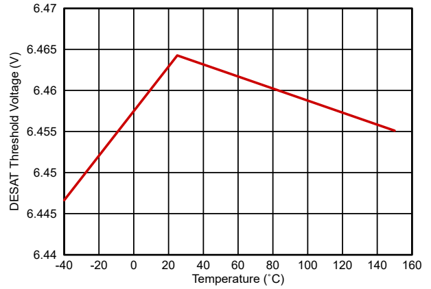
图 5-24. DESAT 阈值与温度间的关系
