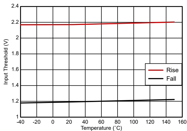
图 5-10. 输入阈值
