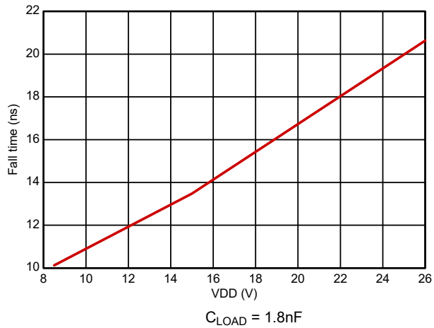
图 5-15. 输出下降时间
