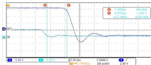
图 7-4. UCC57102Z 下降 ( 关断 ) 传播延迟
