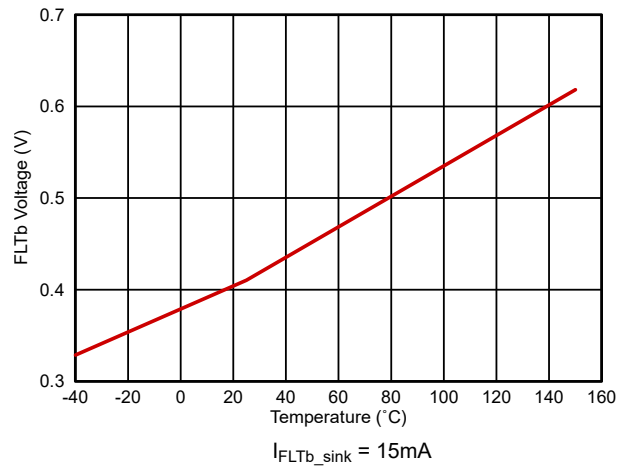
图 5-26. FLTb 与温度间的关系
