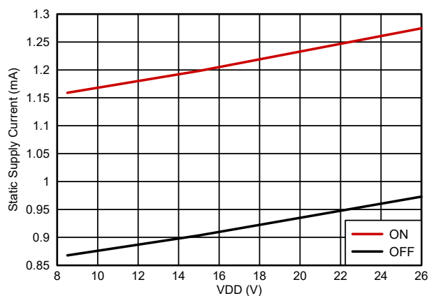
图 5-6. 工作静态电源电流
