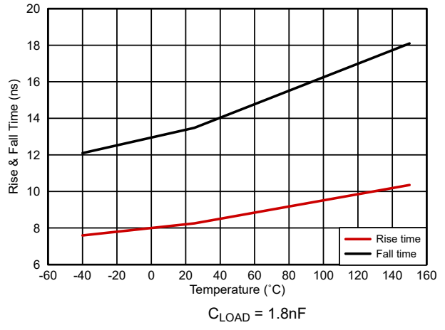
图 5-18. 输出上升和下降时间
