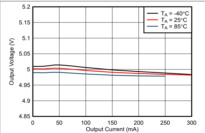
图 6-20. 输出电压调节 ( V_{VCC} ) 与负载电流 ( I_{VCC} ) 间的关系 : V_{CC} = 5.0V , V_{INP} = 5.0V , C_{OUT2} = 22 \mu F
