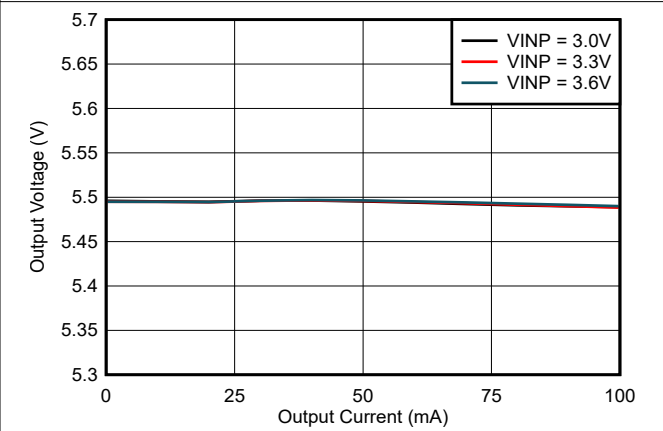
图 6-24. 输出电压调节 ( V_{VCC} ) 与负载电流 ( I_{VCC} ) 间的关系 : V_{CC} = 5.5V , T_A = 25^\circ C , C_{OUT2} = 22 \mu F
