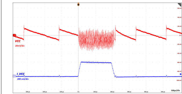
图 6-27. 负载瞬态 : VINP = 5.0V , VCC = 5.0V , C OUT2 = 22 μF , I VCC = 0mA - 300mA - 0mA
