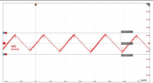
图 6-26. 稳态输出电压纹波 : VINP = 5.0V , VCC = 5.0V , C OUT2 = 22 μF , 300mA 负载
