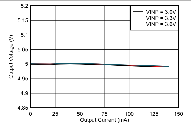
图 6-22. 输出电压调节 ( V_{VCC} ) 与负载电流 ( I_{VCC} ) 间的关系 : V_{CC} = 5.0V , T_A = 25^\circ C , C_{OUT2} = 22 \mu F
