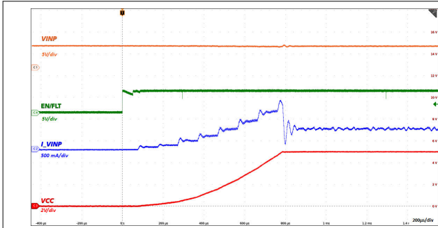
图 6-25. 通过 EN/FLT 从低电平到高电平启动 : VINP = 5.0V , VCC = 5.0V , 18Ω 负载
