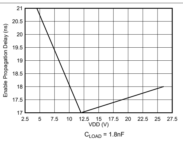
图 5-20. 使能到输出上传传播延迟
