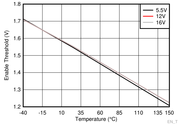
图 6-10. Enable Threshold
