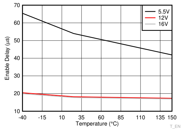
图 6-12. Enable Delay
