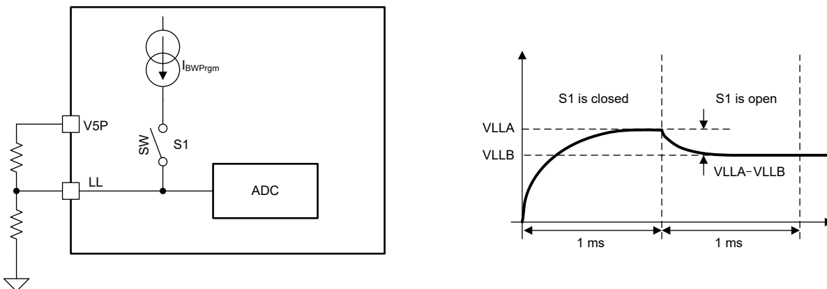
图 7-20. LL 引脚编程
