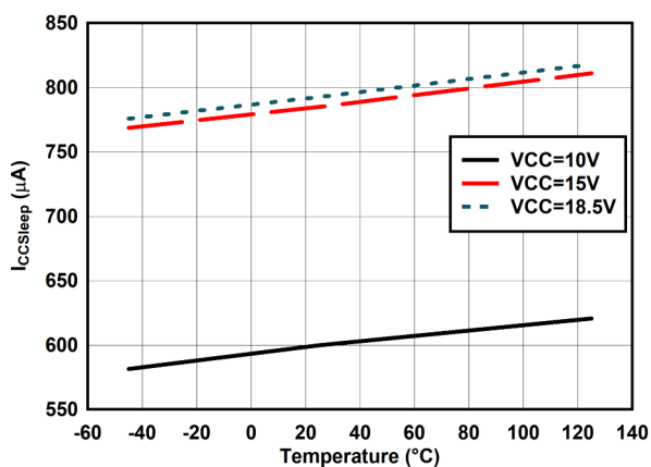
图 6-10. I_{CCSleep} 与温度间的关系
