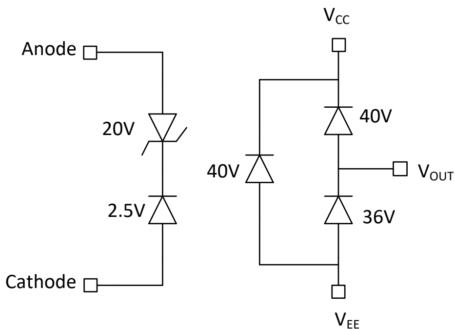
图 9-1. ESD Structure
