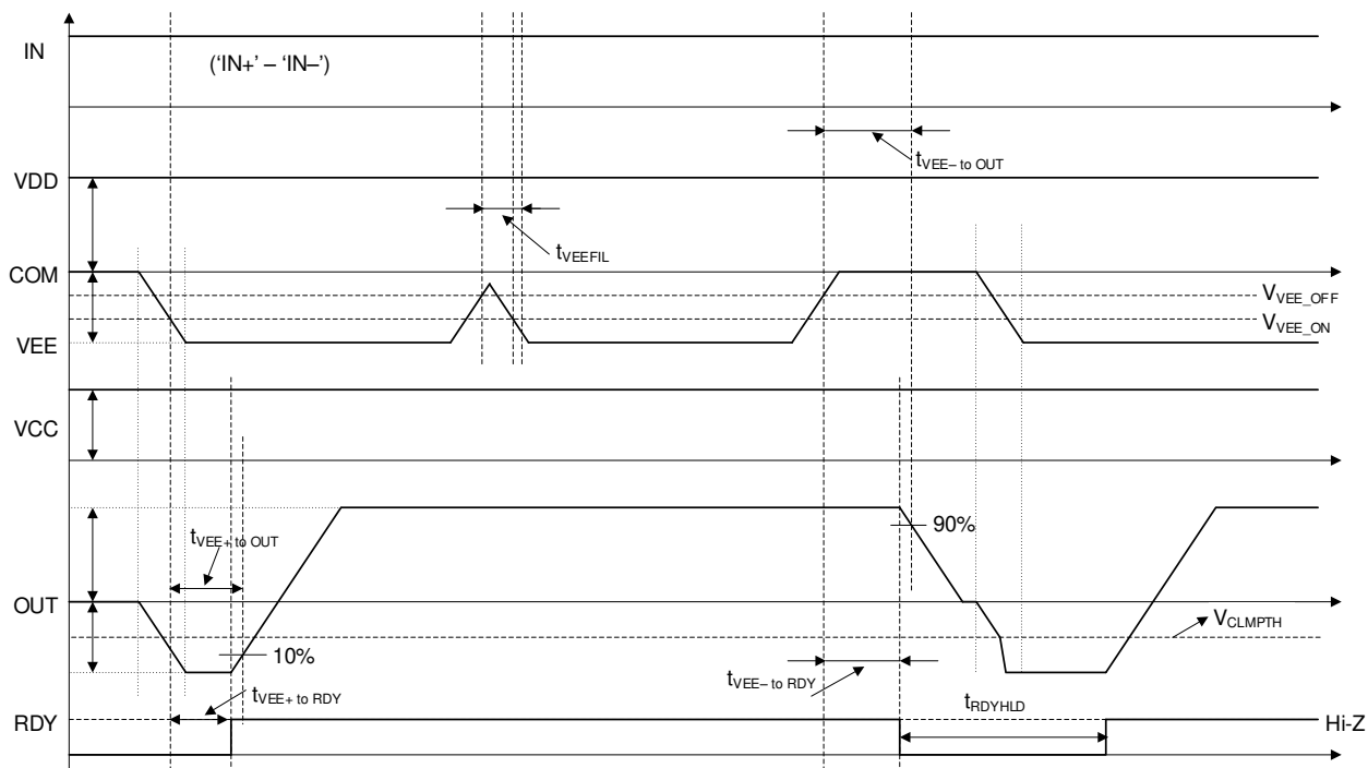
图 6-10. VEE UVLO Protection Timing Diagram
