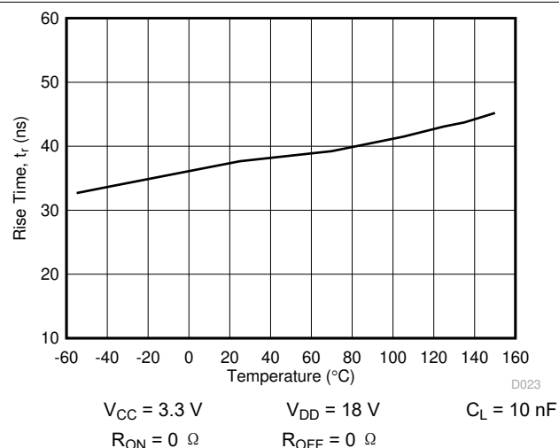
图 5-16. t_r Rise Time vs Temperature
