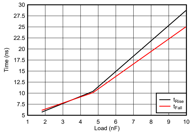
图 5-9. 上升和下降时间与负载间的关系 ( V_{DD} = 15V )
