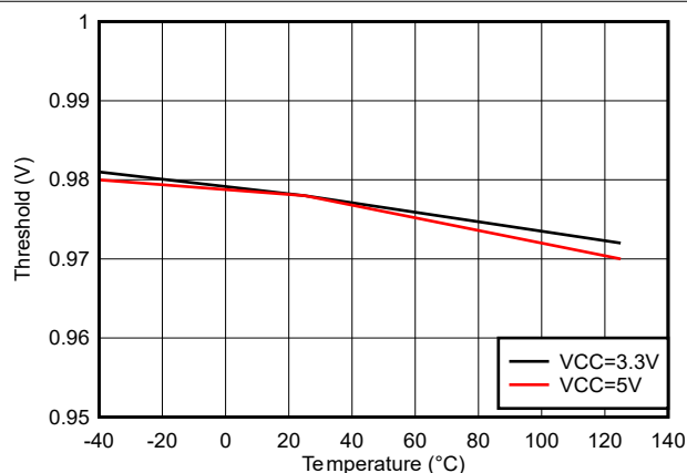
图 5-19. IN/EN 低阈值
