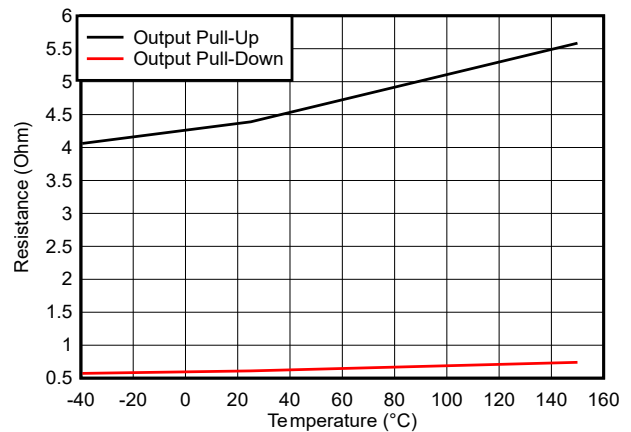
图 5-10. 输出电阻与温度之间的关系
