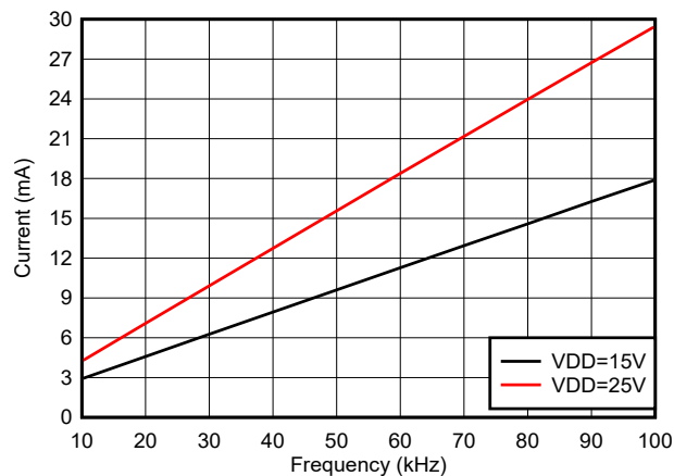
图 5-5. 每通道电流消耗 ( I_{VDDA/B} ) 与频率之间的关系 (10nF 负载, V_{DD} = 15V 或 25V )
