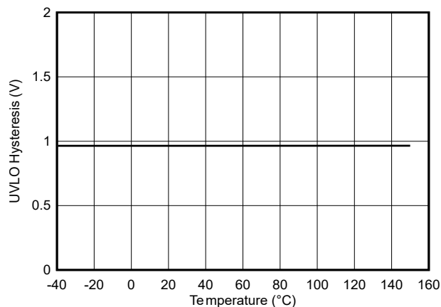
图 5-17. VDD 12V UVLO 迟滞与温度之间的关系
