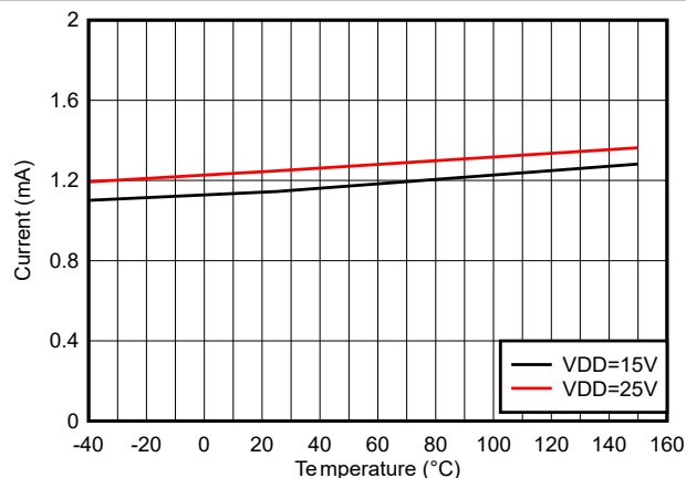
图 5-7. 每通道 ( I_{VDDA/B} ) 静态电源电流与温度之间的关系 (无负载, 低电平输入, 无开关)
