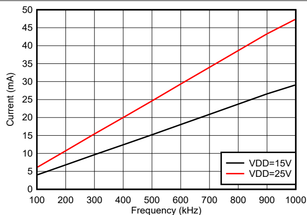
图 5-4. 每通道电流消耗 ( I_{VDDA/B} ) 与频率之间的关系 (1nF 负载, V_{DD} = 15V 或 25V )
