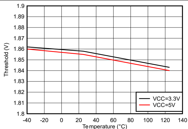
图 5-20. IN/EN 高阈值
