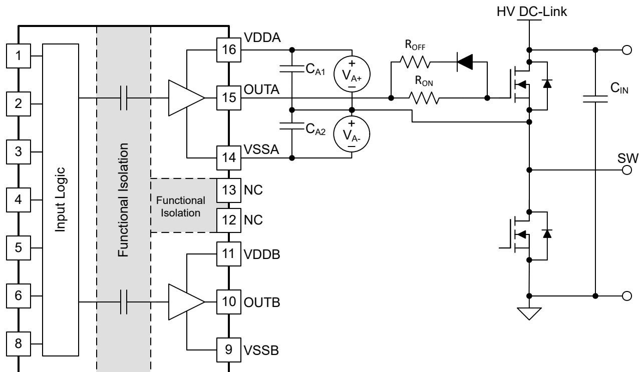
图 8-3. 利用两个 LSO 偏置电源生成负偏置
