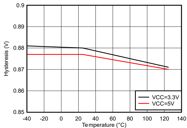
图 5-18. IN/EN 迟滞与温度之间的关系
