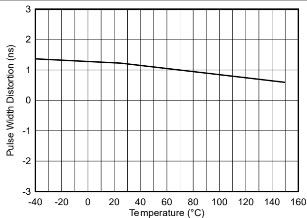
图 5-13. 脉宽失真度与温度之间的关系
