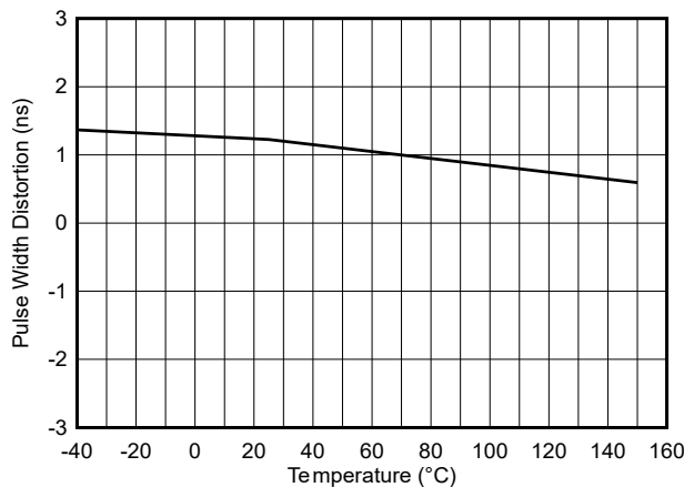
图 5-13. 脉宽失真度与温度之间的关系
