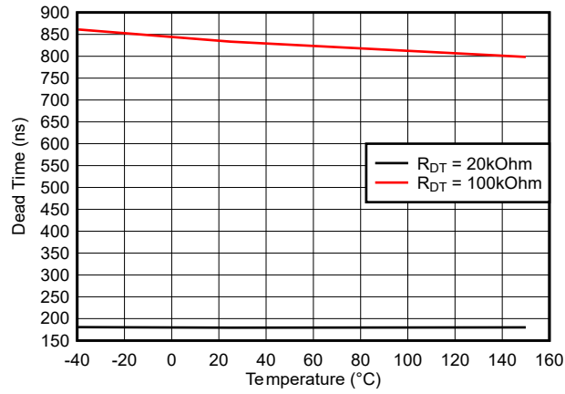
图 5-21. 死区时间与温度之间的关系 ( R_{DT} = 20k\Omega 和 100k\Omega )
