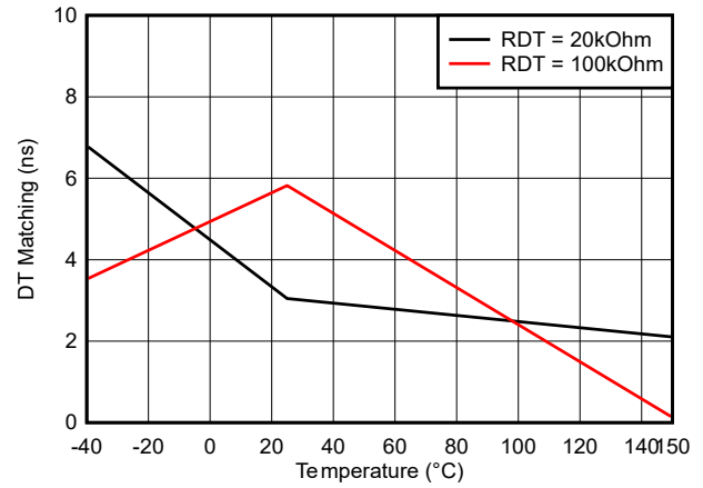
图 5-22. 死区时间匹配与温度之间的关系 ( R_{DT} = 20k\Omega 和 100k\Omega )
