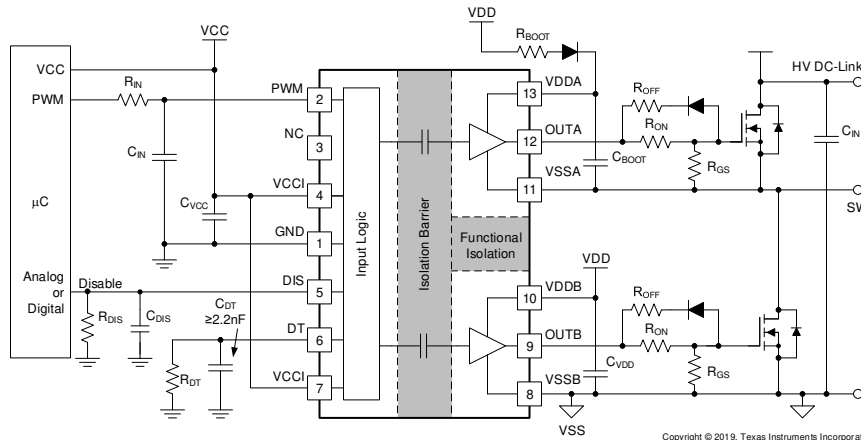
功能方框图
