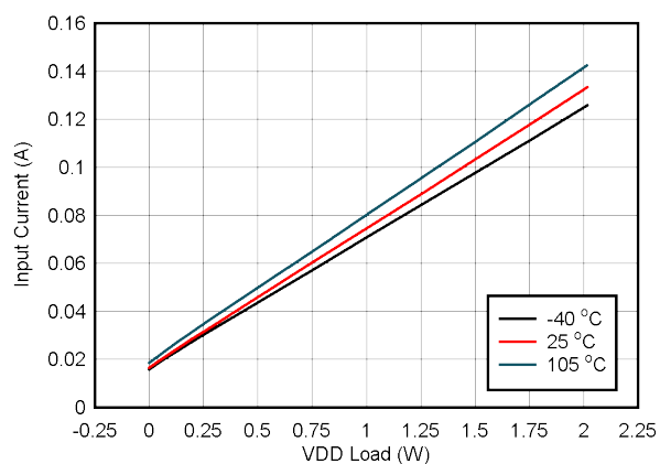
图 6-20. Input Current vs Load on V_{DD-VEE} : V_{IN} = 27\text{ V} , V_{DD-VEE} = 25\text{ V} , V_{COM-VEE} = 5\text{ V} , No Load on V_{COM-VEE}
