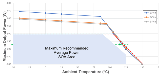
图 6-4. SOA Derating Curves: V_{DD-VEE} = 25\text{ V} , V_{COM-VEE} = 5\text{ V} , No Load
