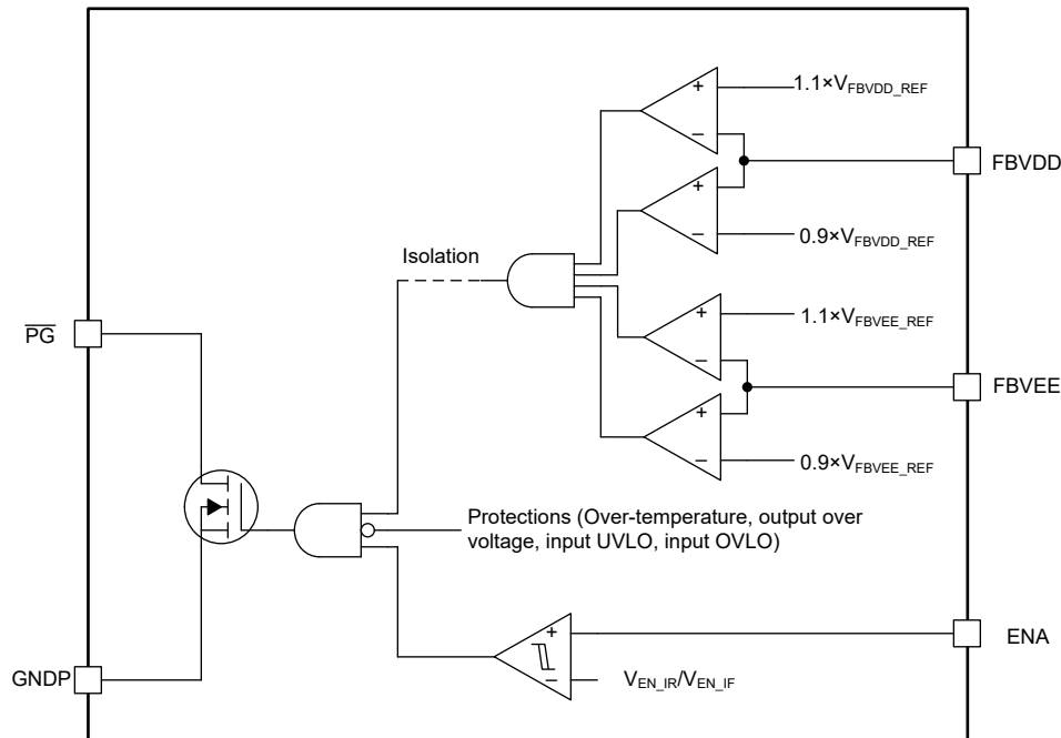
图 7-7. \overline{\text{PG}} Pin Logic
