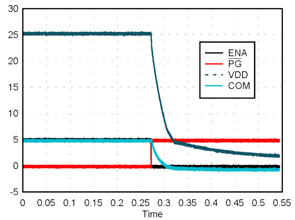
图 6-6. Shutdown: V_{IN} = 24\text{ V} , V_{DD-VEE} = 25\text{ V} , V_{COM-VEE} = 5\text{ V} , No Load
