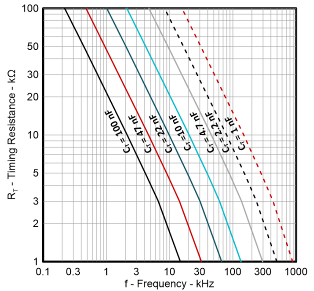
图 6-10. 时序电阻 R_{RT} 与频率间的关系
