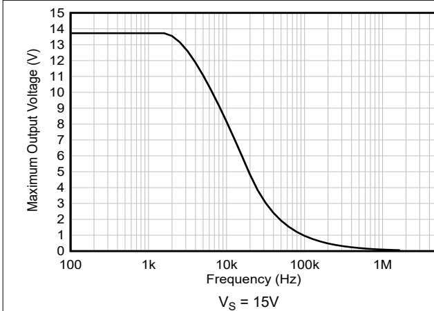
图 5-9. 最大输出电压与频率间的关系 (新裸片)
