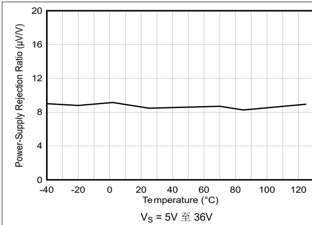
图 5-7. 电源抑制比与温度间的关系 (新裸片)
