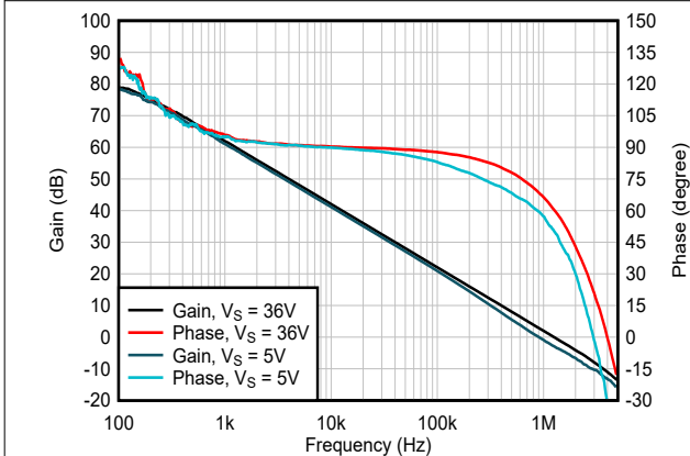
图 5-11. 开环增益和相位与频率间的关系 (新裸片)
