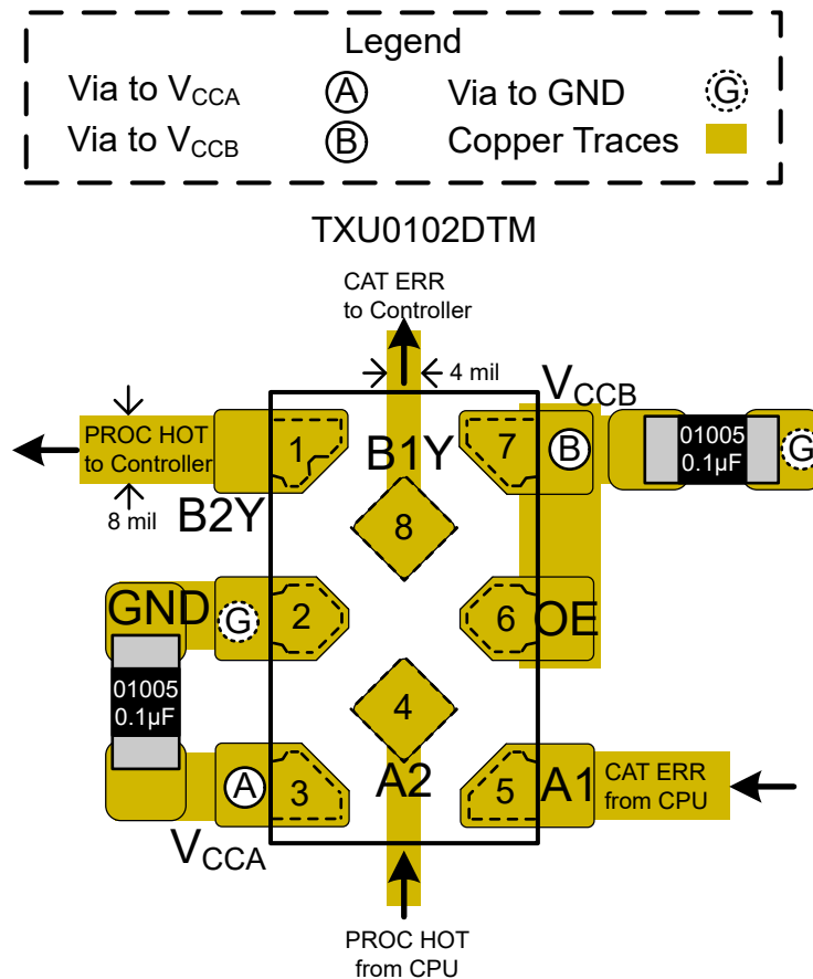
图 12-1. Layout Example – TXU0102
